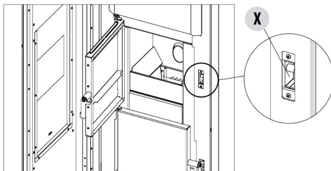
Fig. 81 - Chiusura sportello
