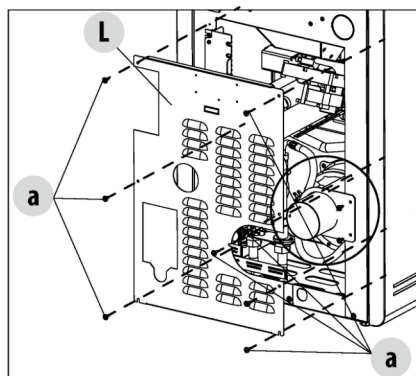
Fig. 72 - Pannello posteriore
