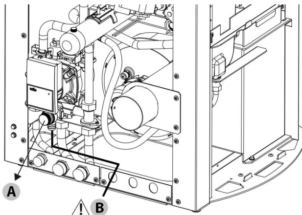
Fig. 57 - Valvola di scarico
