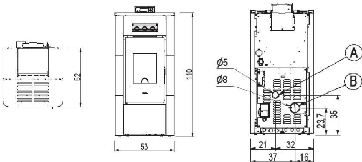
Fig. 17 - EGEA IDRO 18 - 24
