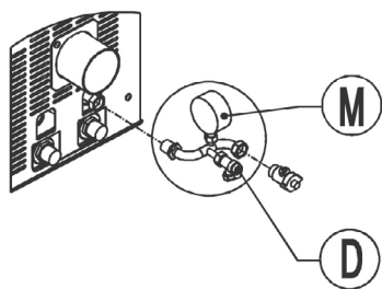
Fig. 58 - Terminale con rubinetto di caricamento (D) e manometro (M)
