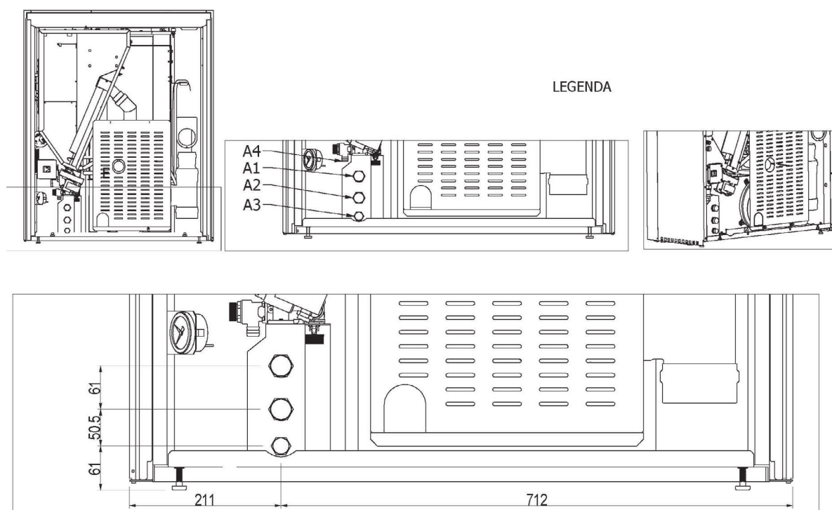
Fig. 56 - Schema allacciamento
