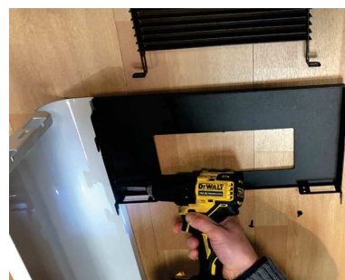
Fig. 25 - Fissare il pannello al montante
