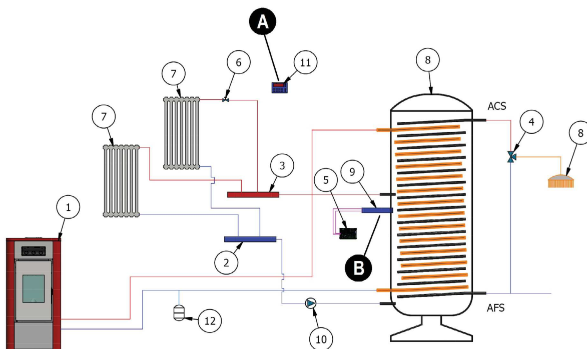
Fig. 66 - Configurazione 5
