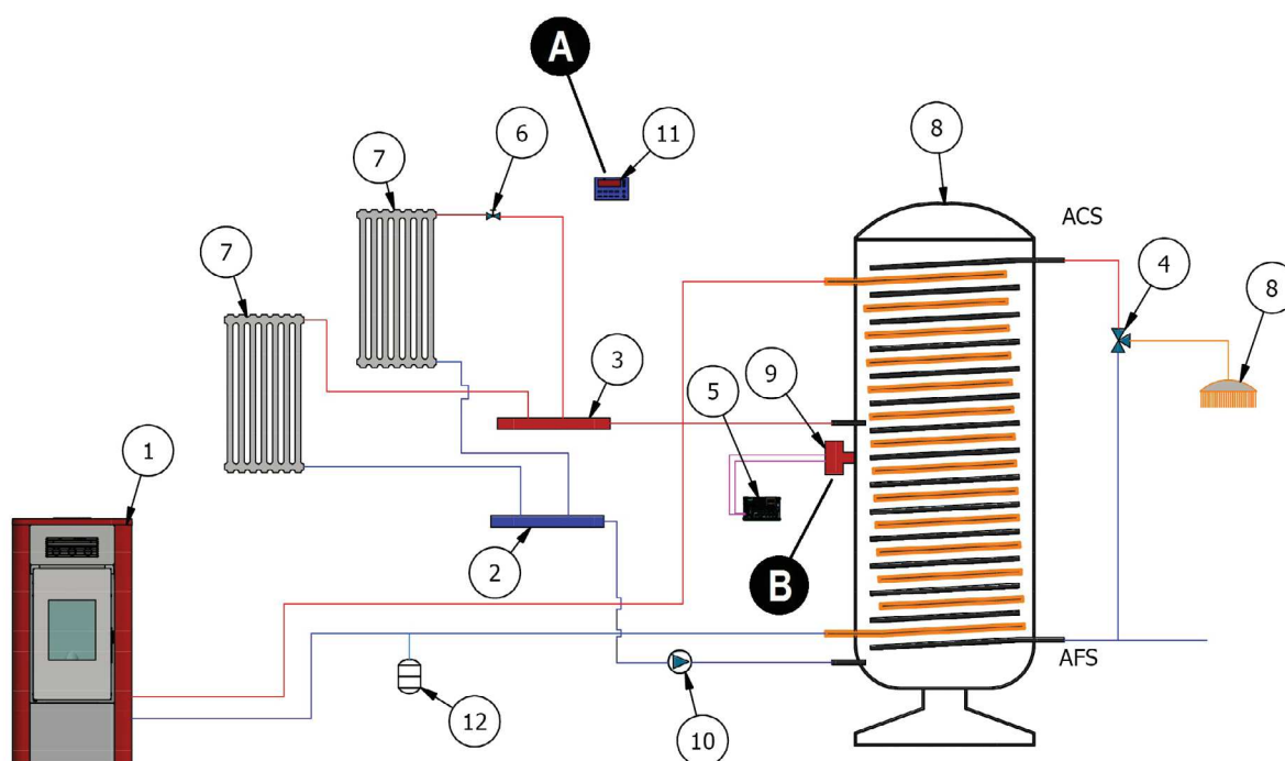
Fig. 65 - Configurazione 4
