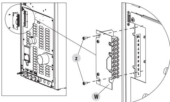
Fig. 70 - Collegamenti
