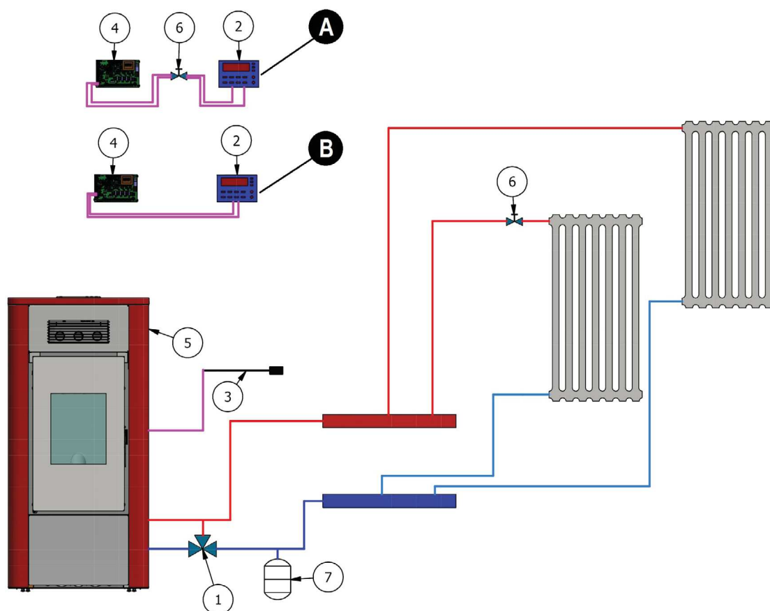
Fig. 61 - Configurazione 1
