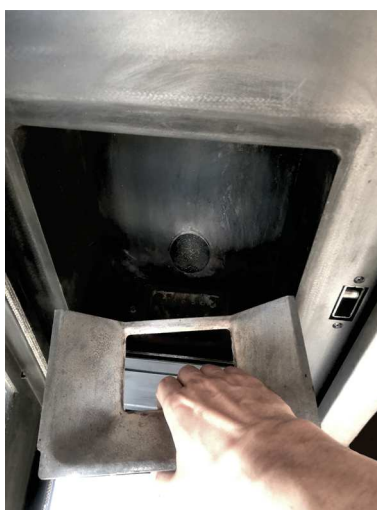
Fig. 85 - Aspirare cenere
