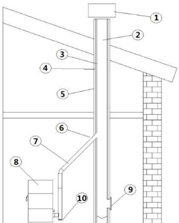
Fig. 5 - Componenti camino
