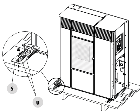
Fig. 3 - Rimozione staffe di fissaggio
