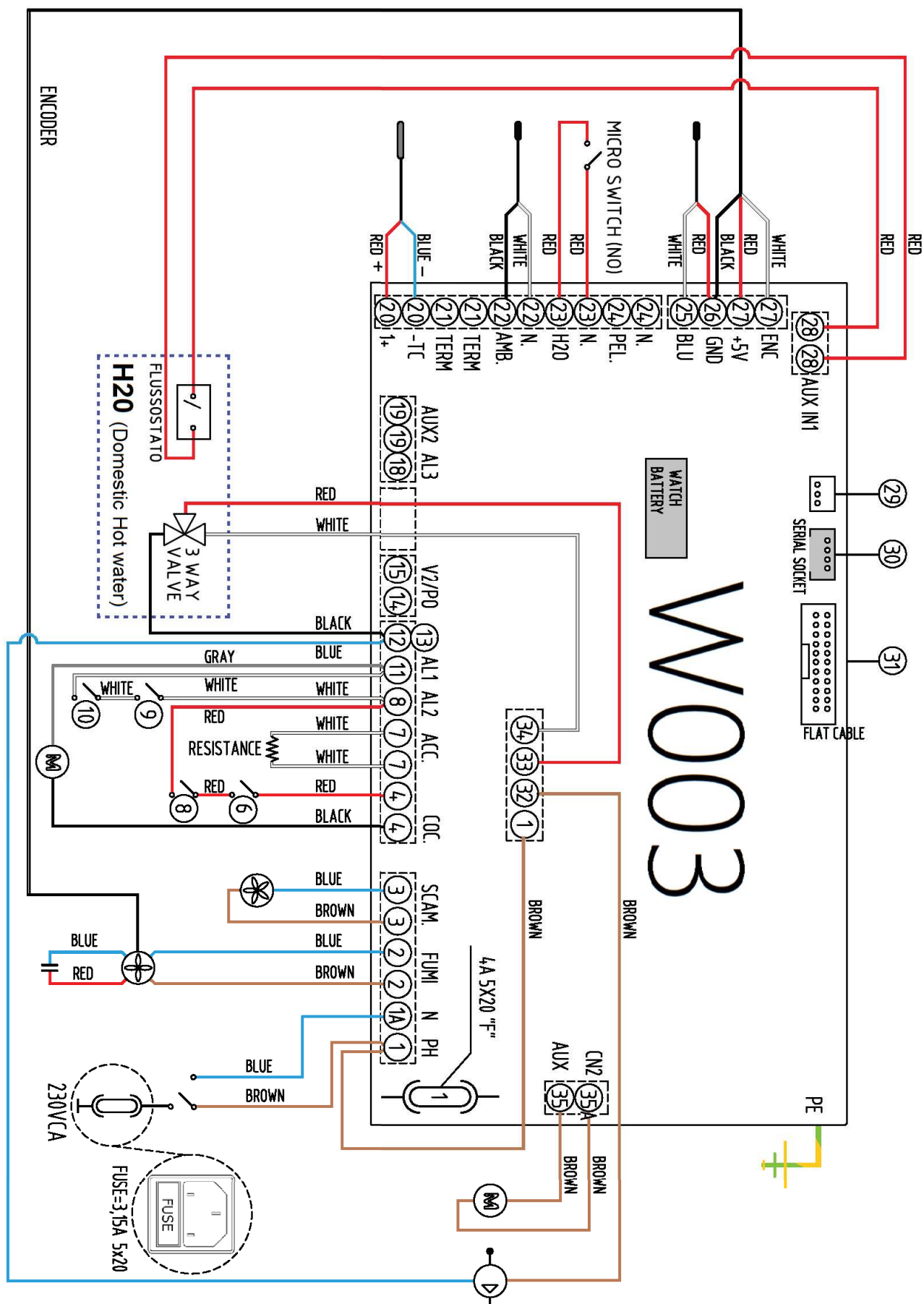
Fig. 104 - Scheda elettronica senza kit sanitario
