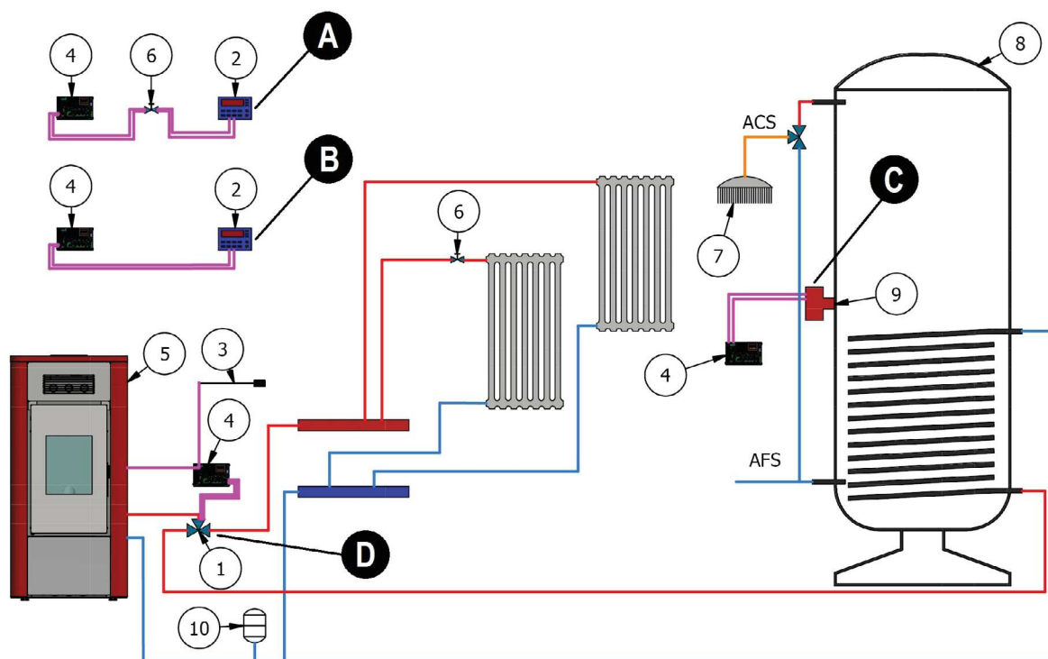
Fig. 63 - Configurazione 2b
