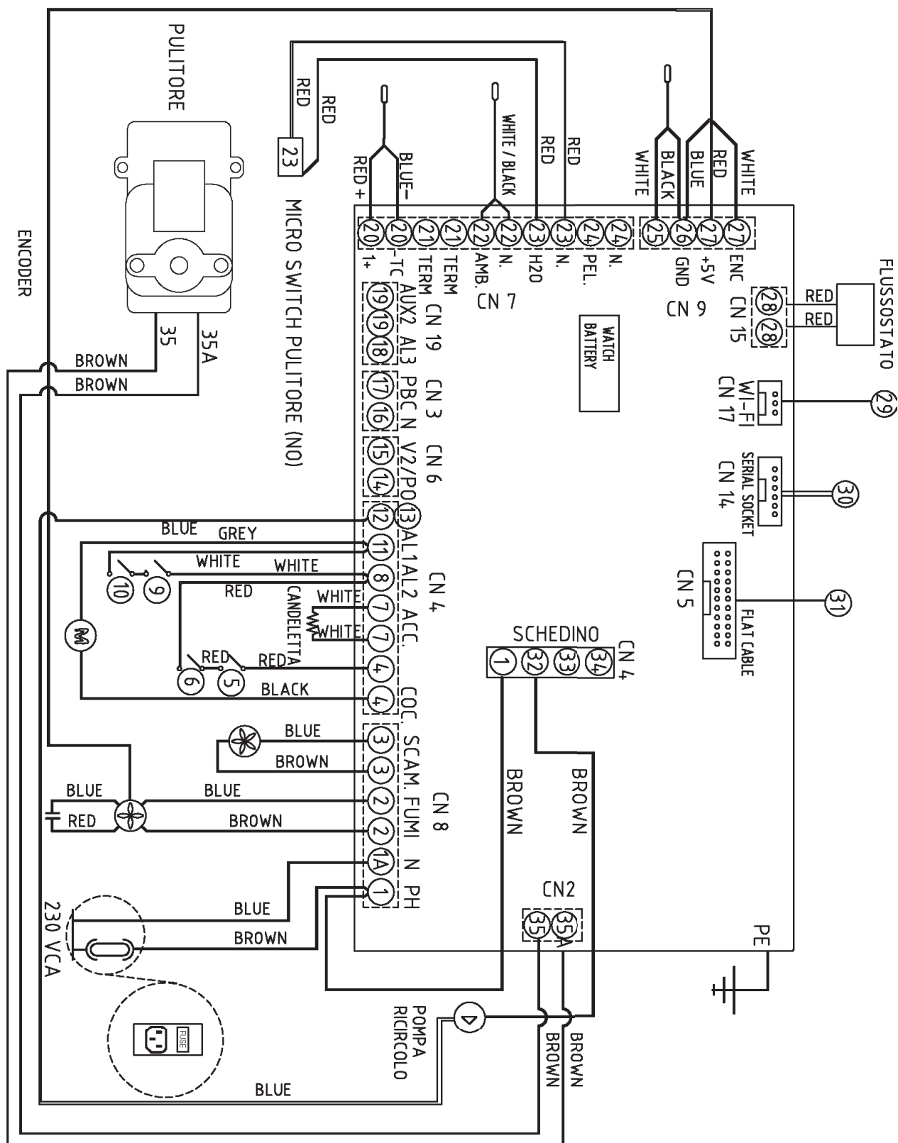
Fig. 105 - Scheda elettronica con kit sanitario
