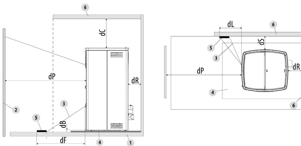
Fig. 15 - Distanze di sicurezza da materiale combustibile
