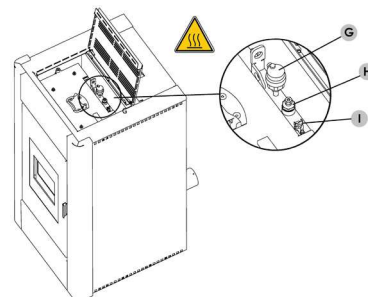
Fig. 60 - Valvola di sfiato manuale posta sotto il top (Idro Prince 3 30-30 H2O)
