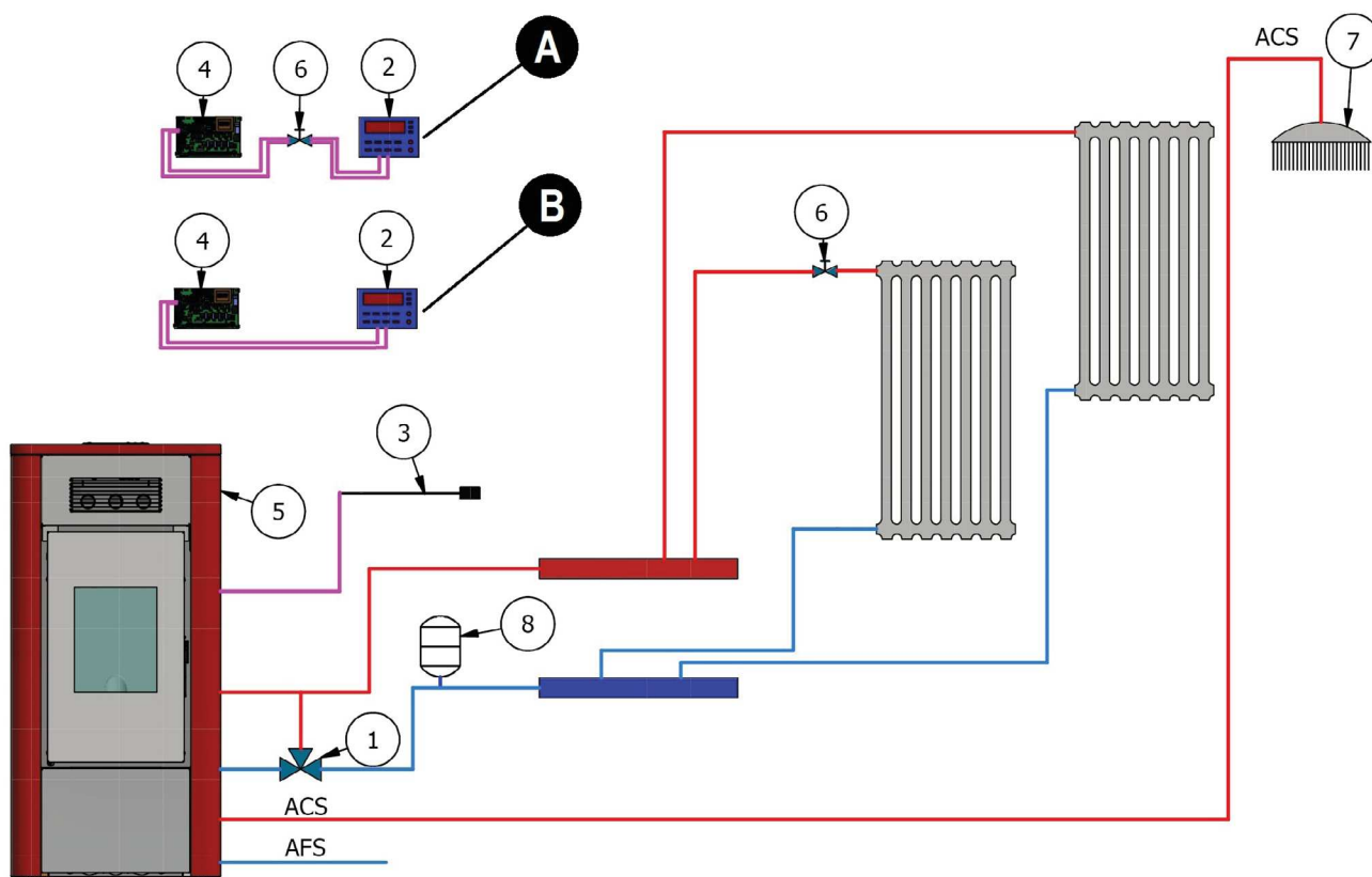
Fig. 62 - Configurazione 2a
