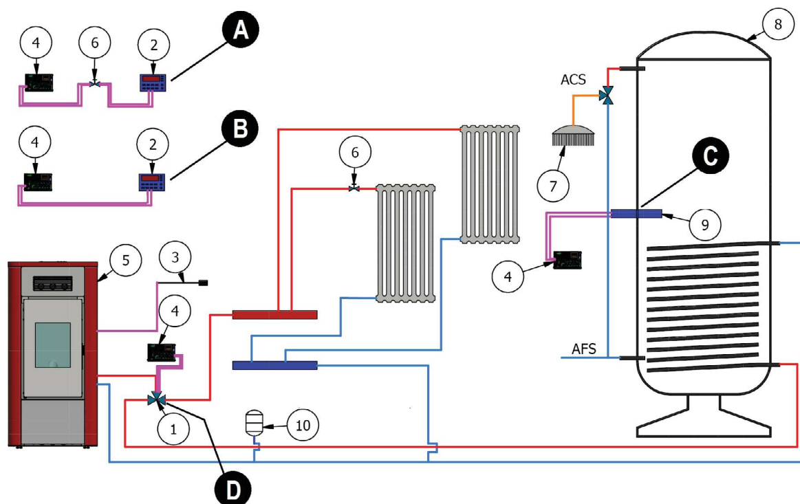
Fig. 64 - Configurazione 3
