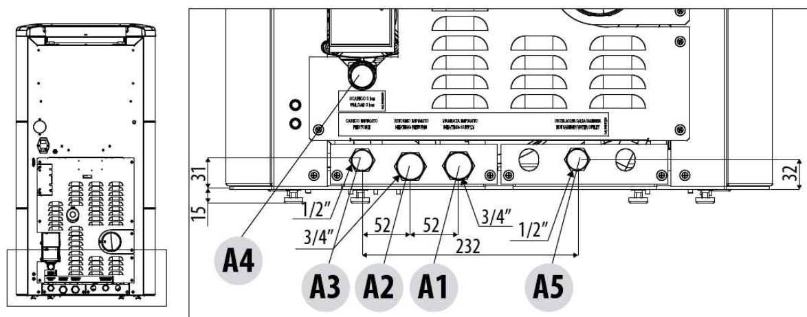
Fig. 55 - Schema allacciamento con ACS
