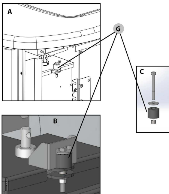
Fig. 89 - Gommino
