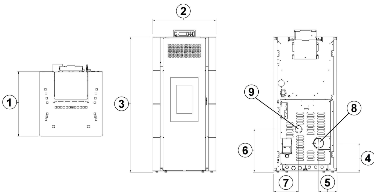
Fig. 18 - MIRA 18/24 - TESIS 18/24
