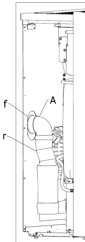
Fig. 52 - Uscita fumi posteriore
