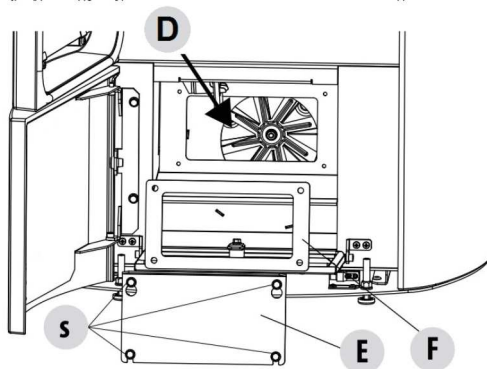
Fig. 80 - Pulizia vano inferiore
