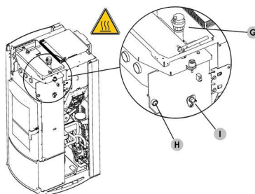
Fig. 59 - Valvola di sfiato manuale posta sotto il top (Idro Prince 3 16-23-23 H2O, Aquos 3 16-23-23 H2O, Idron 16-22 Airtight, Hidrofire 22.8)
