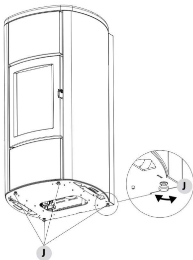
Fig. 4 - Regolazione piedini
