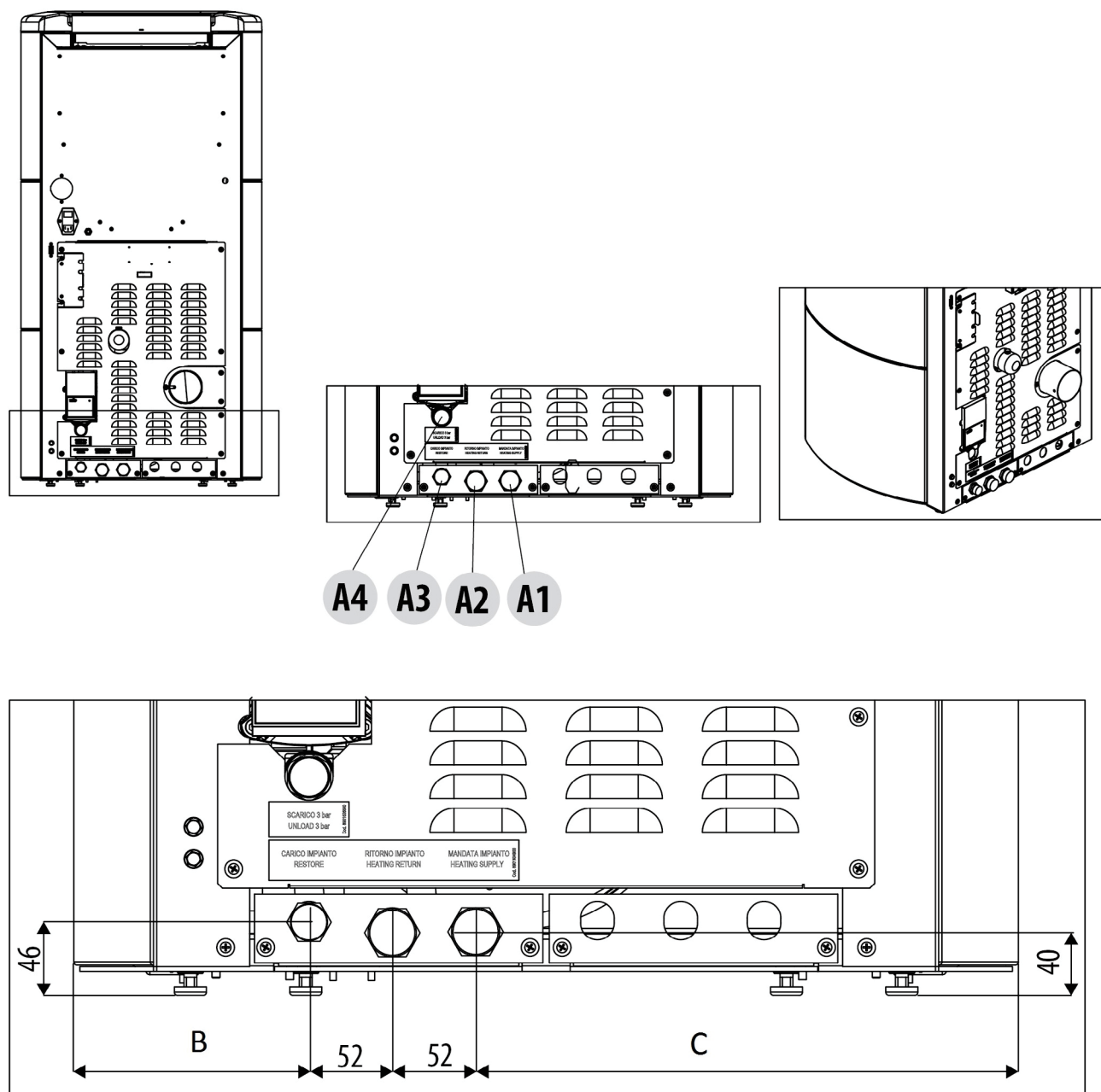
Fig. 54 - Schema allacciamento
