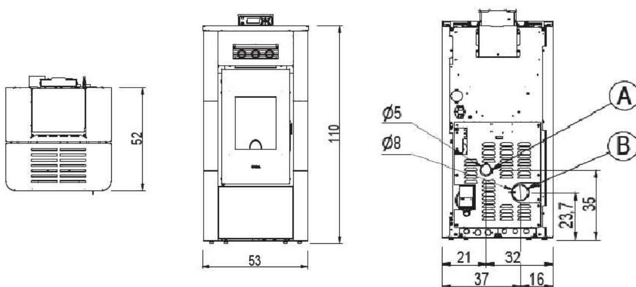
Fig. 16 - RIVER IDRO 18 - 24
