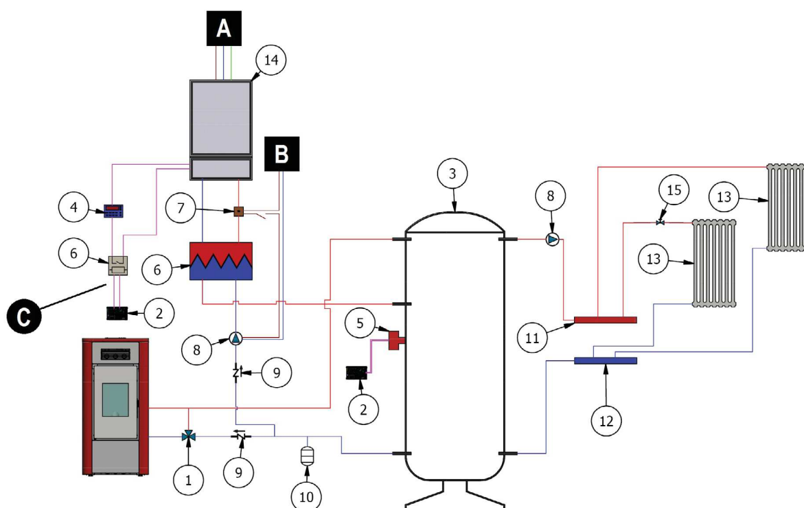
Fig. 67 - Configurazione con boiler e caldaia murale di soccorso
