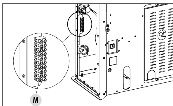
Fig. 71 - Collegamenti
