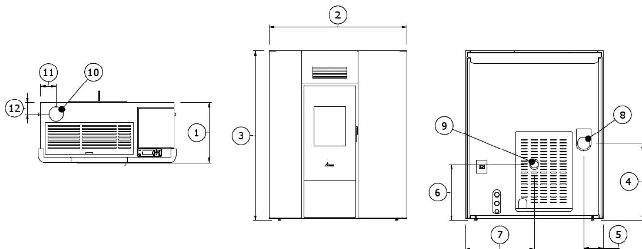
Fig. 19 - MAYA IDRO 18 - 24
