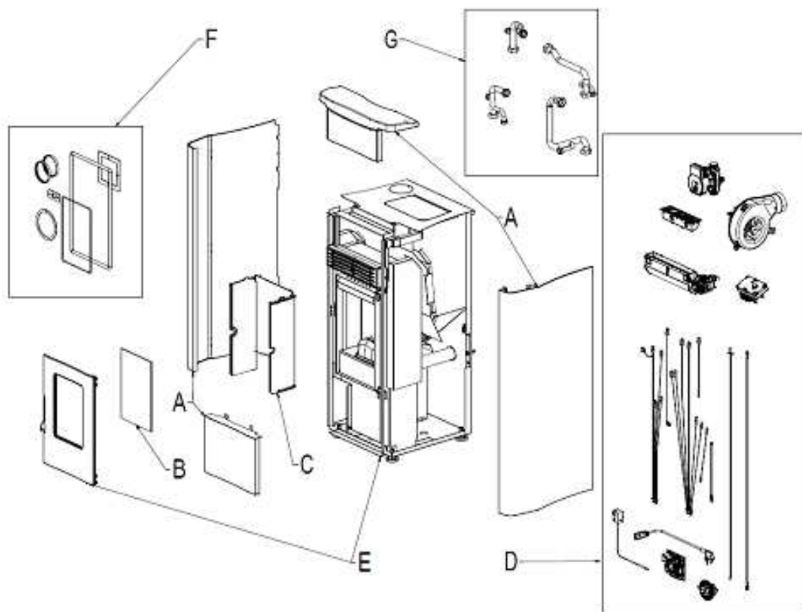
Fig. 1 - Geëxplodeerde tekening
