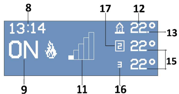
Fig. 6 - Display
