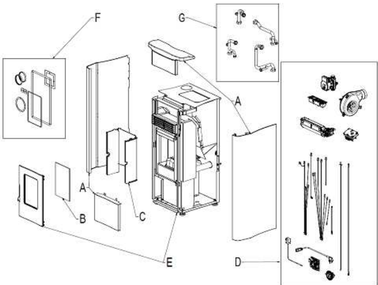
Fig. 1 - Dibujo explotado
