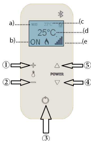
Fig. 26 - Fernsteuerung mit Thermostat
