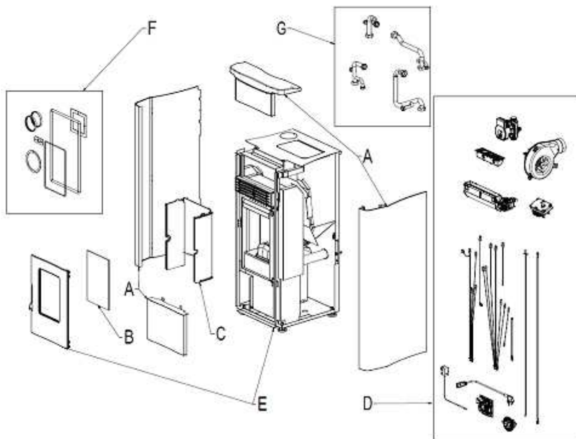
Fig. 1 - Explosionszeichnung
