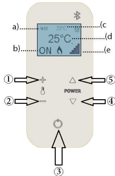
Fig. 26 - Télécommande avec thermostat
