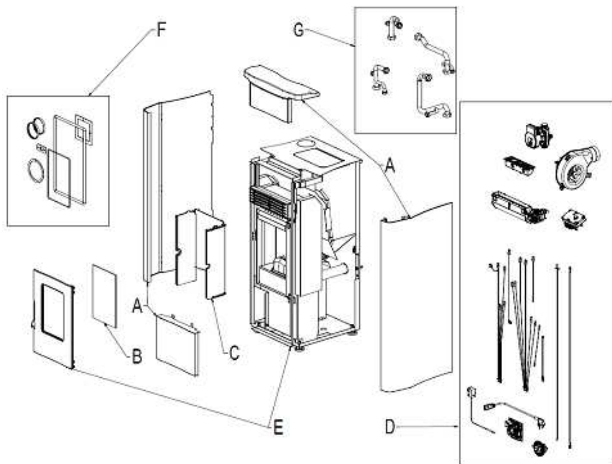
Fig. 1 - Dessin éclaté
