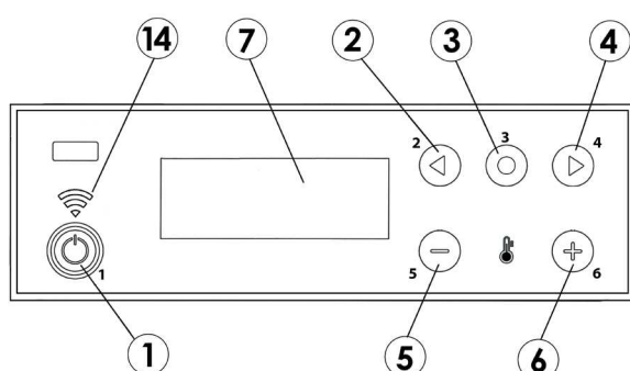
Fig. 5 - Tableau de controle (wi-fi)
