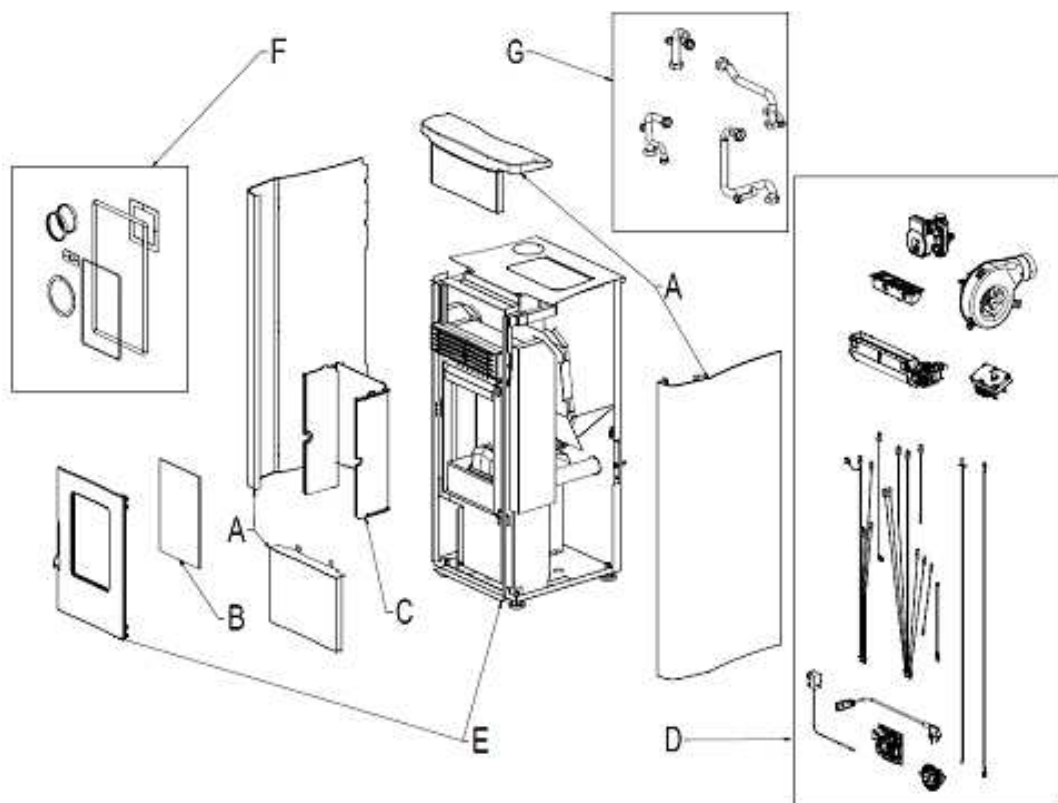
Fig. 1 - Explosionszeichnung
