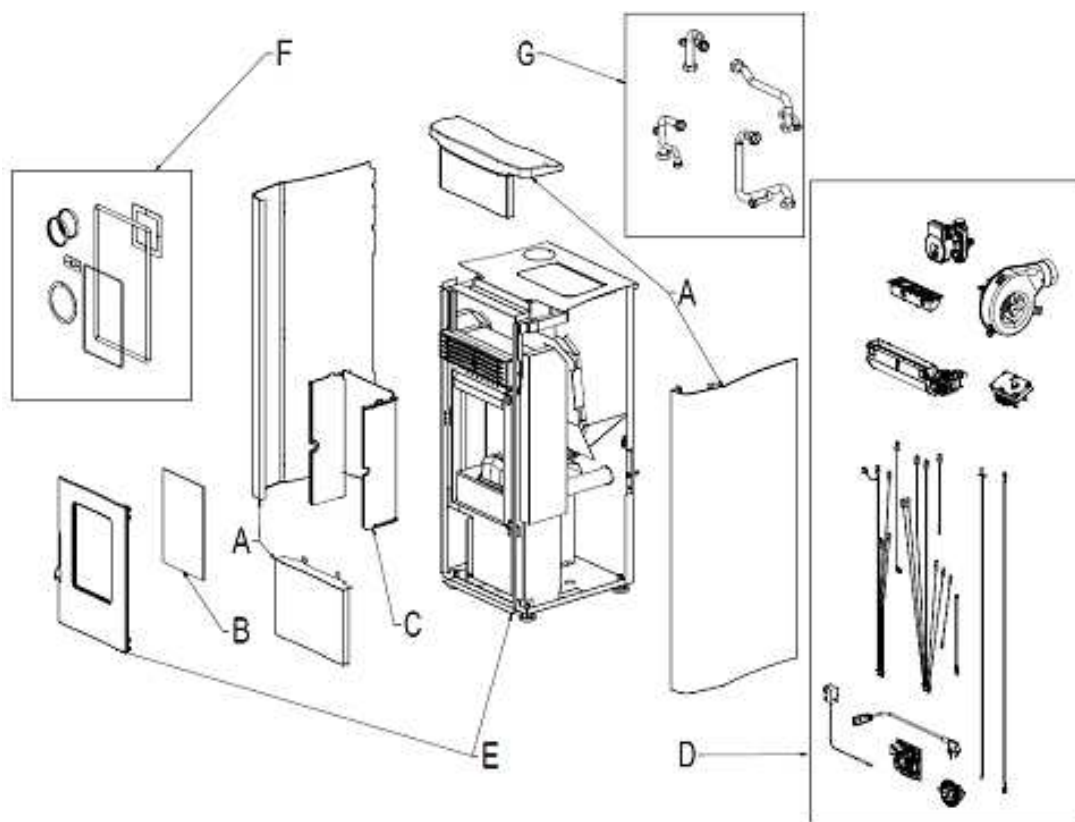
Fig. 1 - Esploso
