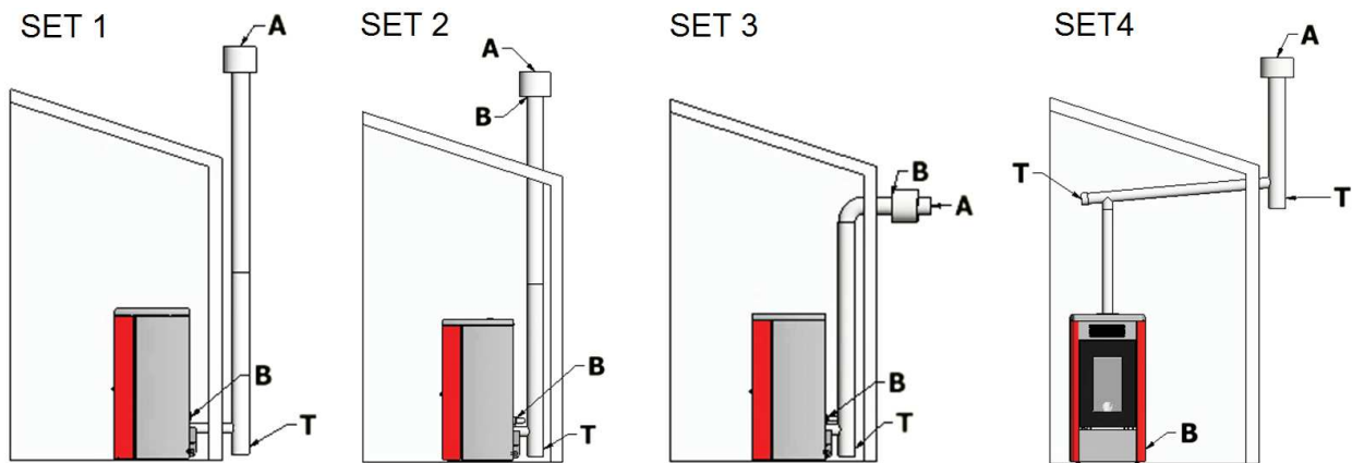
Fig. 20 - Esempi Set
