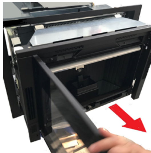
Fig. 25 - Maschinenkörper entnehmen
