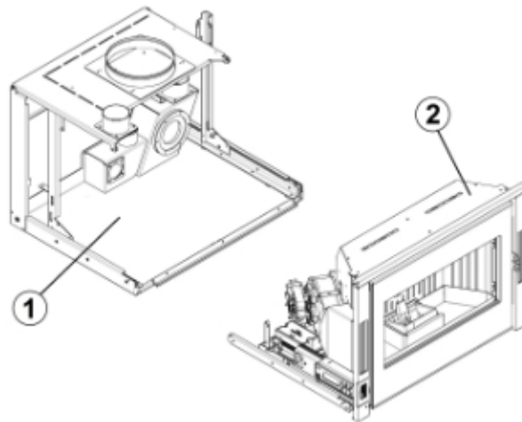
Fig. 23 - Struktur + Maschinenkörper
