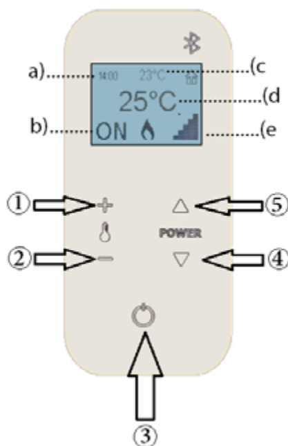
Fig. 38 - Fernsteuerung mit Thermostat
