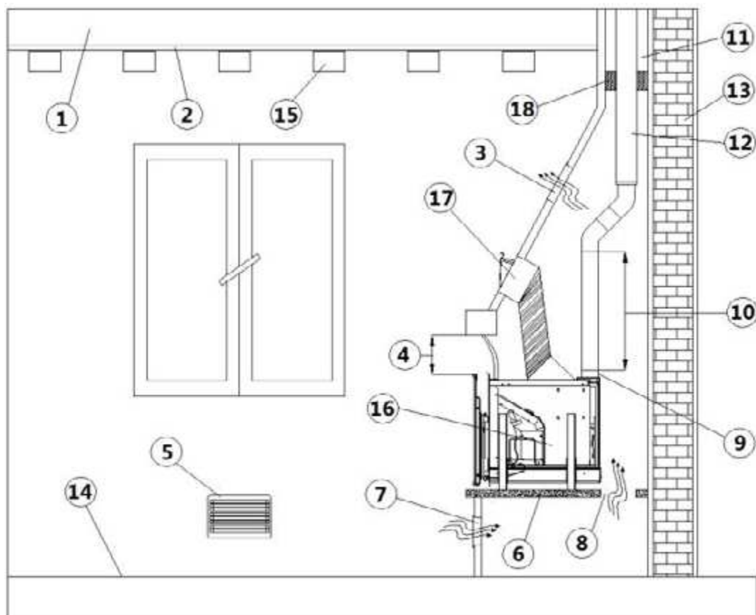
Fig. 26 - Installatie in een bestaande haard
