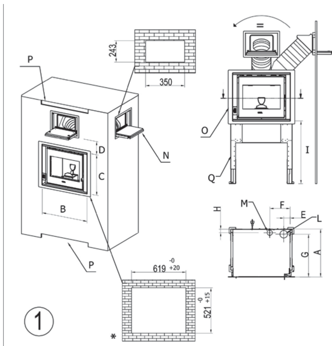
Fig. 14 - PONENTE - ZENITH met laaddeur + frame
