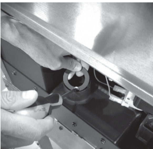
Fig. 79 - Verwijder de ring
