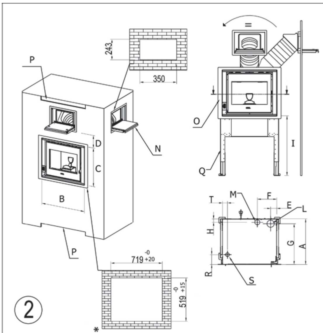
Fig. 15 - ZEN - ZEFIRO met laaddeur + frame
