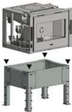
Fig. 36 - Bevestig het inbouwelement boven
