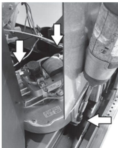
Fig. 96 - Verwijdering van de schroeven - Reiniging 1
