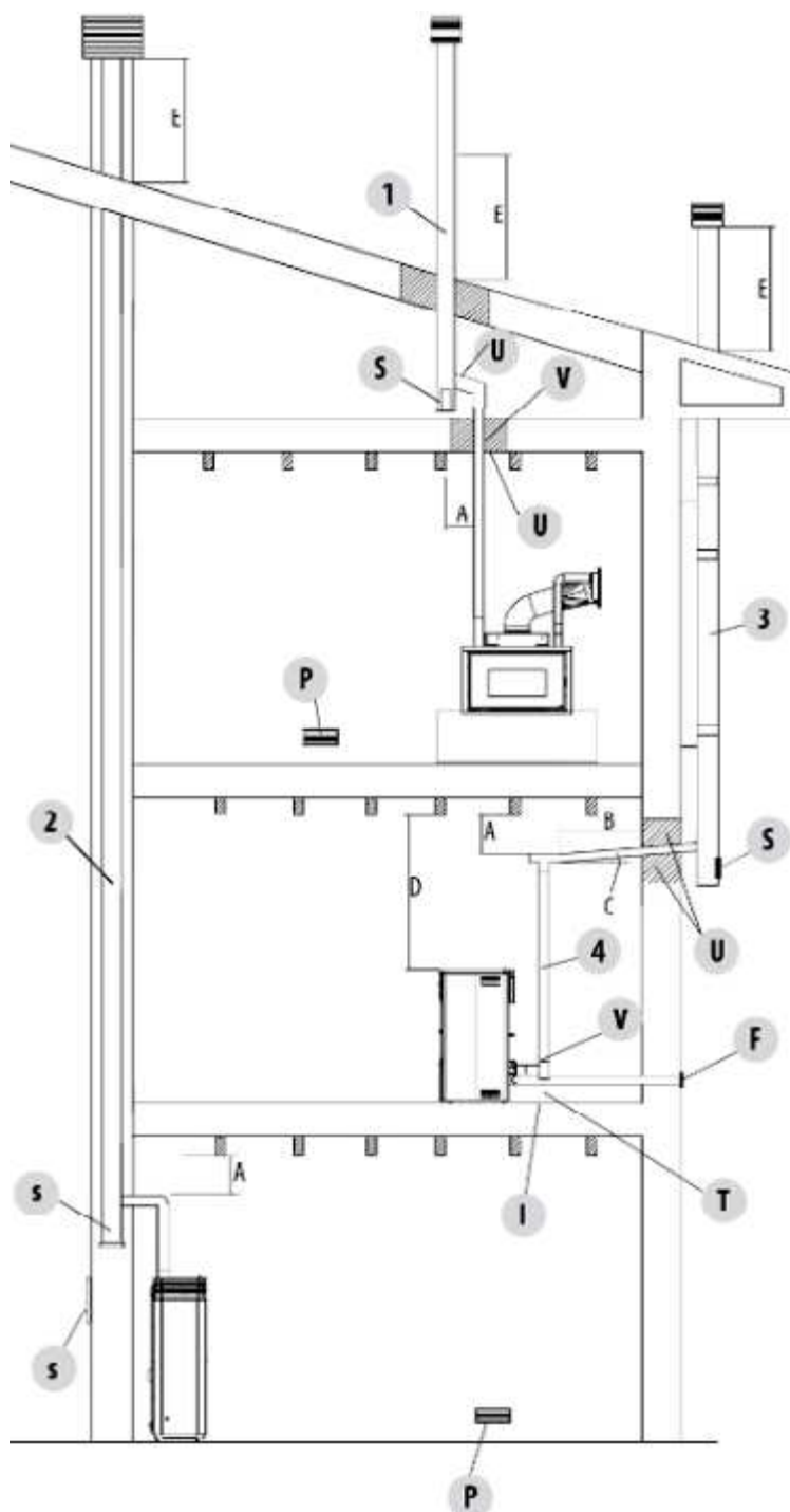
Fig. 12 - Rookkanaal
