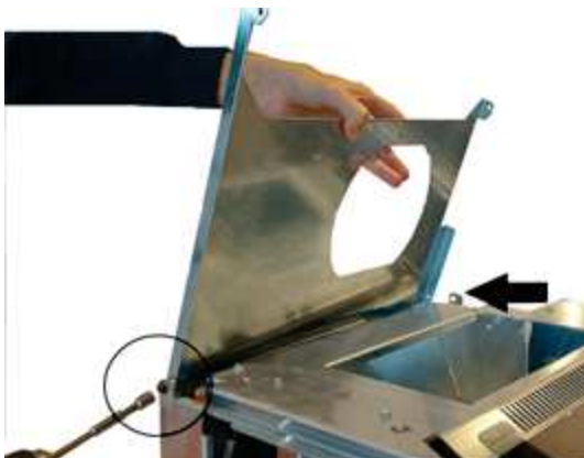
Fig. 51 - Verwijder het deksel 1
