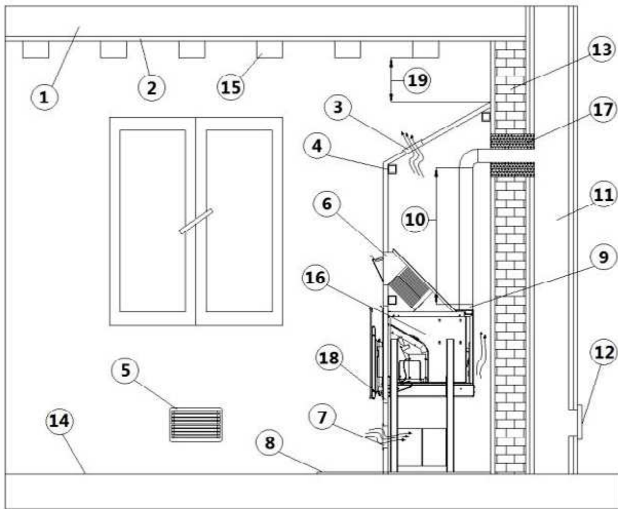
Fig. 25 - Installatie met bekleding
