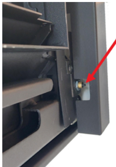
Fig. 41 - Handmatige reset bevindt zich aan de voorkant, rechts (ZEN - ZEFIRO 2026)
