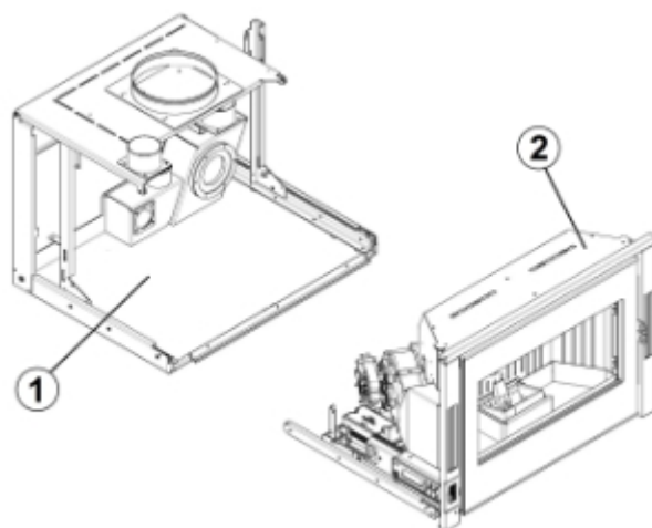
Fig. 23 - Structuur + machineromp
