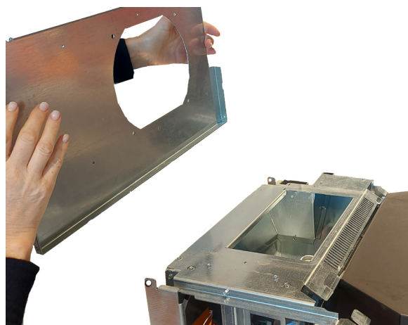
Fig. 52 - Rimuovi coperchio 2
