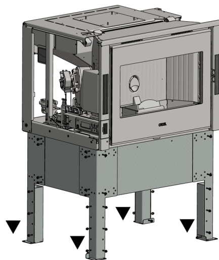
Fig. 37 - Fissare la struttura al pavimento e muro
