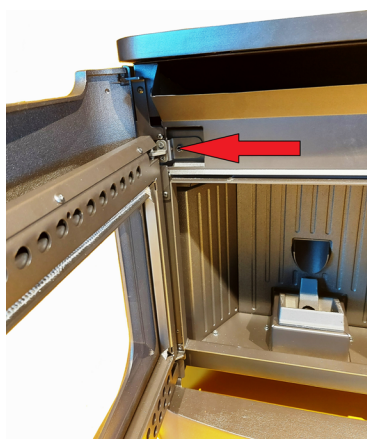
Fig. 28 - Regolazione porta PONENTE
