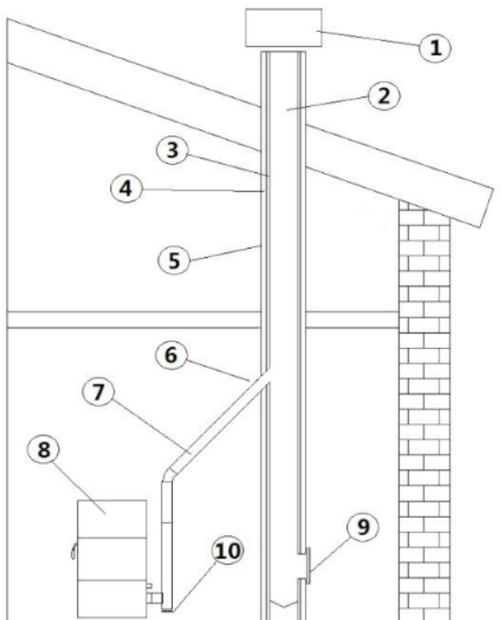
Fig. 2 - Componenti camino
