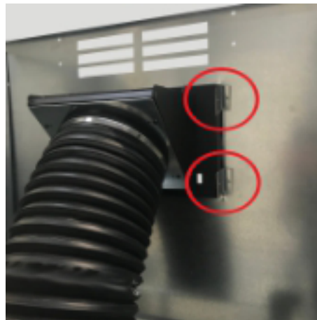
Fig. 71 - Fissaggio interno botola
