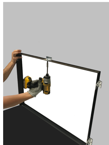
Fig. 78 - Fissaggio posteriore 2
