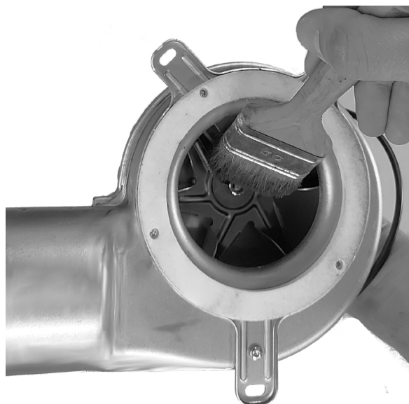
Fig. 97 - Pulizia 2
