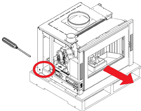
Fig. 1 - Rimozione viti
