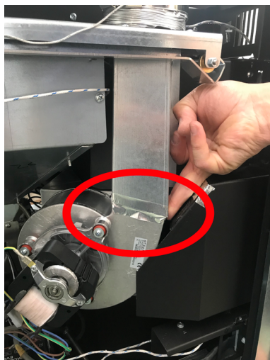
Fig. 47 - Sigillare con nastro adesivo in alluminio
