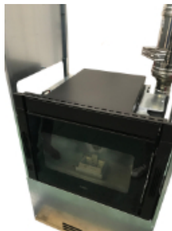
Fig. 61 - Inserimento inserto
