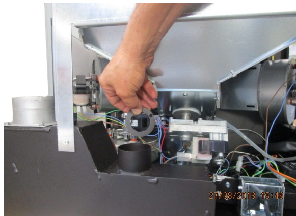
Fig. 33 - Rimozione anello 2
