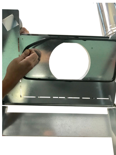
Fig. 54 - Rimozione guarnizione
