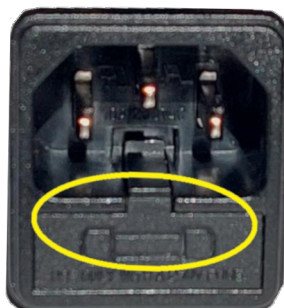
Fig. 114 - Sportellino con i fusibili da rimuovere
