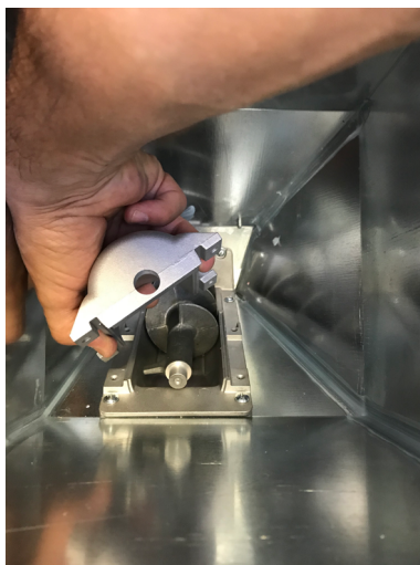
Fig. 88 - Rimozione guscio
