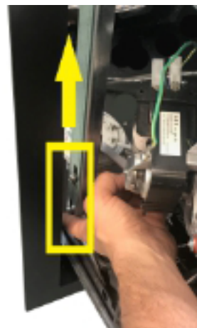
Fig. 22 - Sollevare piastrina di bloccaggio
