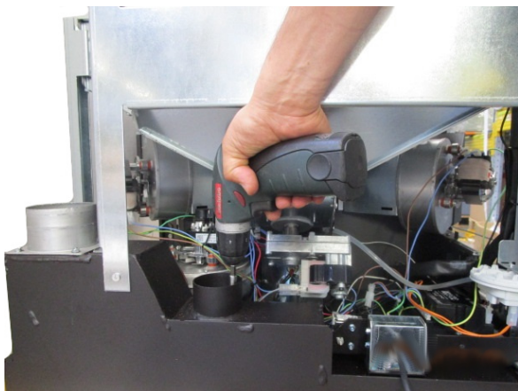
Fig. 32 - Rimozione anello 1
