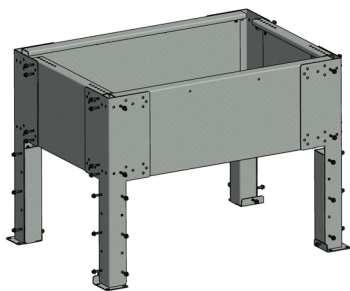
Fig. 34 - Assemblare gambe
