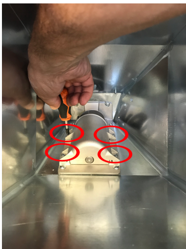
Fig. 87 - Rimozione viti
