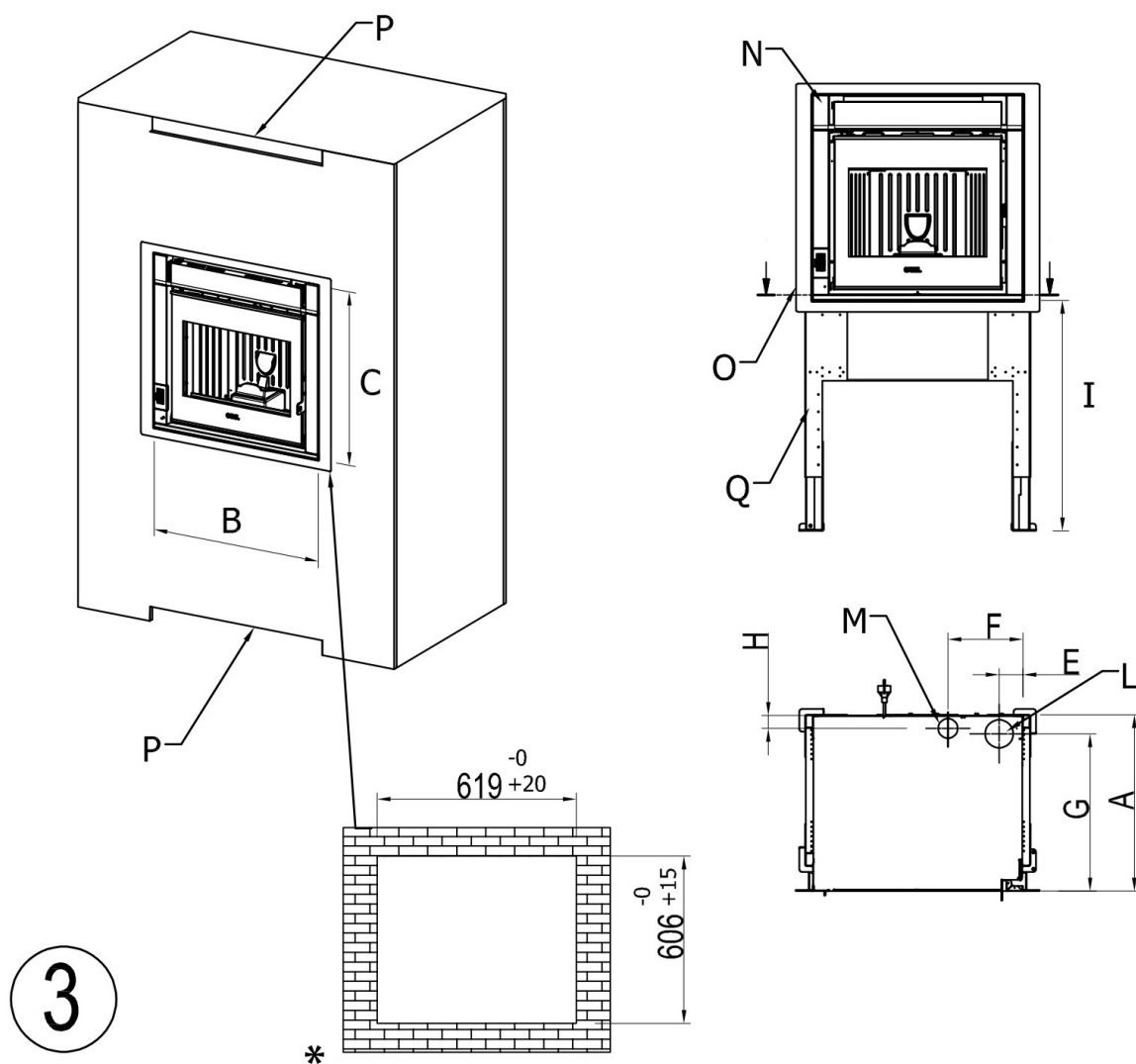
Fig. 16 - PONENTE - ZENITH cassette+cornice
