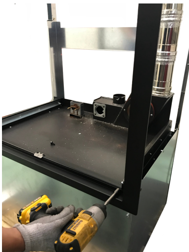
Fig. 76 - Fissaggio frontale
