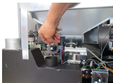
Fig. 10 - Fase 2
