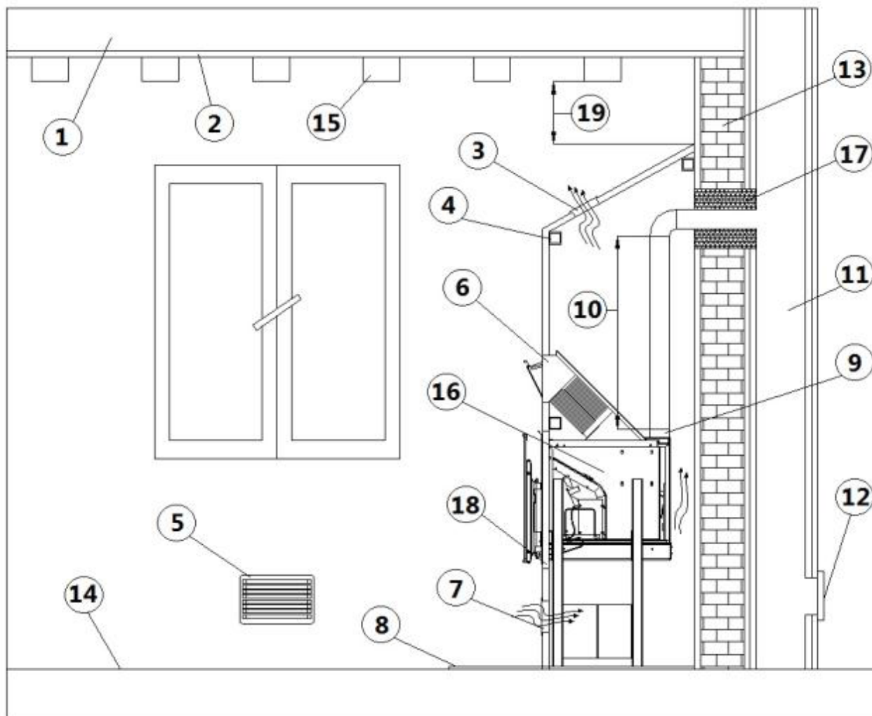
Fig. 25 - Installazione con rivestimento
