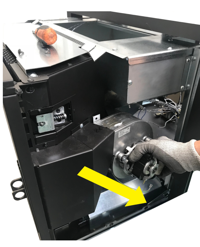
Fig. 95 - Rimuovere ventilatore
