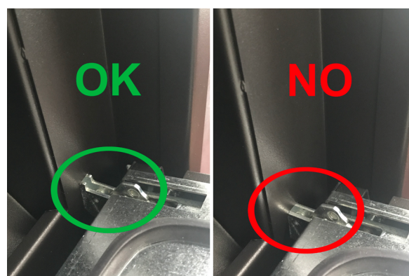
Fig. 73 - Aggancio corretto della cerniera
