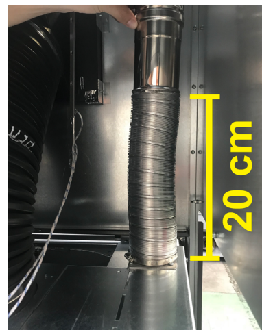
Fig. 49 - Collegamento tubo flessibile (vista posteriore dell'inserto)
