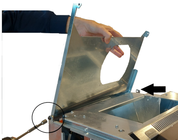
Fig. 51 - Rimuovi coperchio 1
