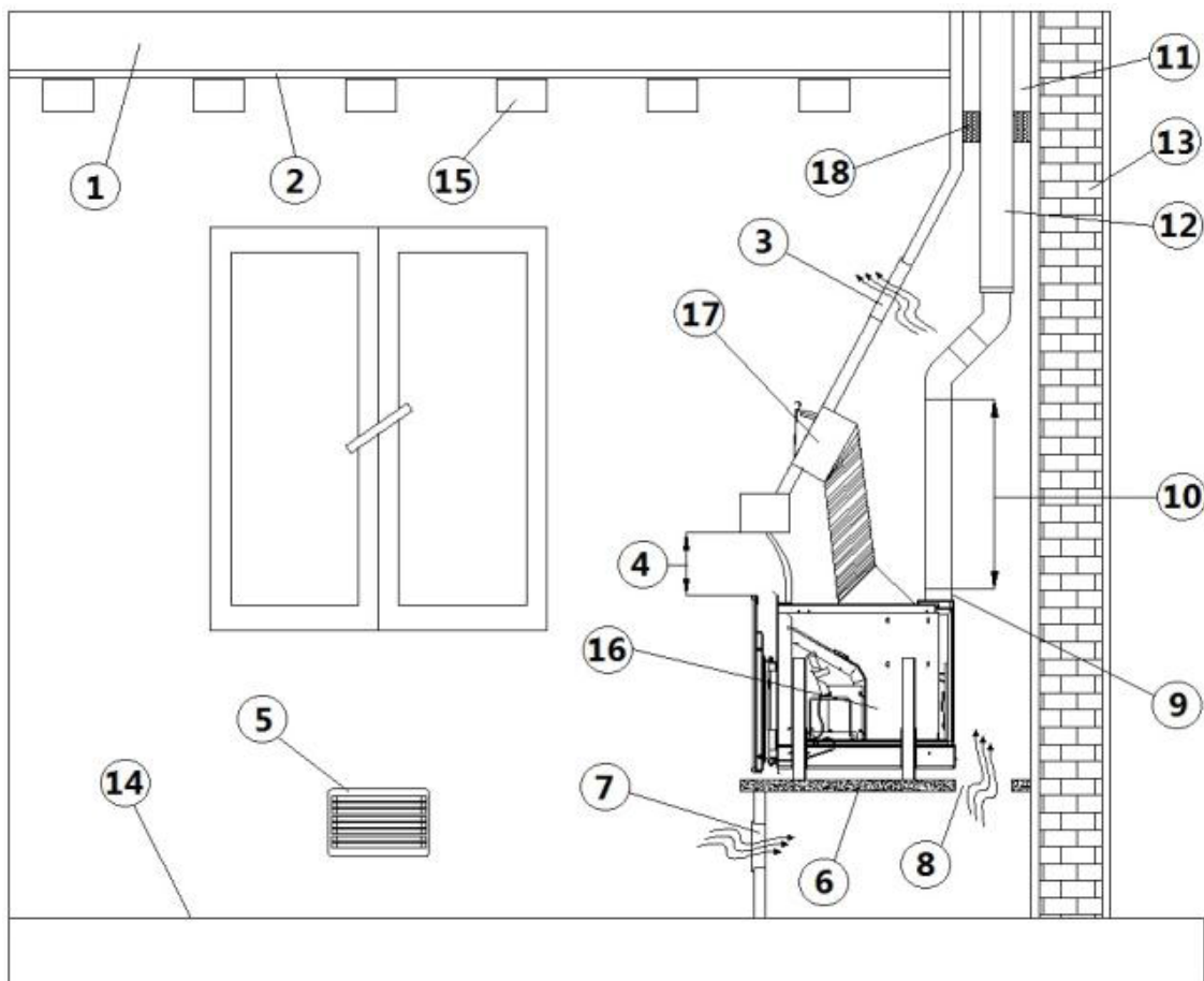
Fig. 26 - Installazione su caminetto esistente
