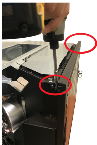
Fig. 53 - Rimozione profilo superiore
