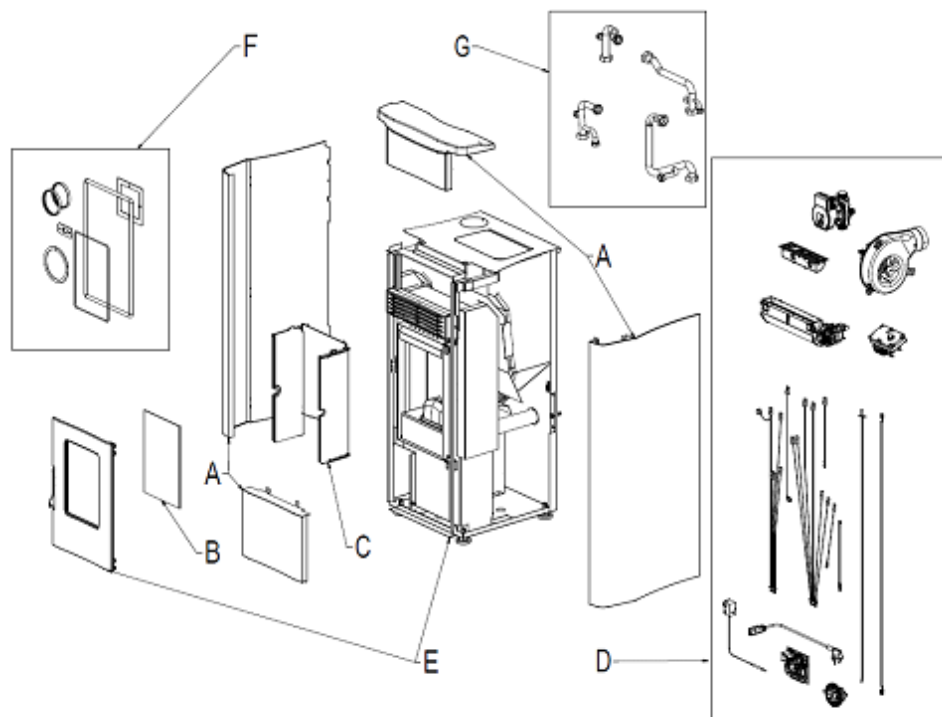
Fig. 1 - Esploso
