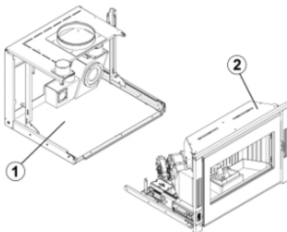
Fig. 23 - Struttura + corpo macchina
