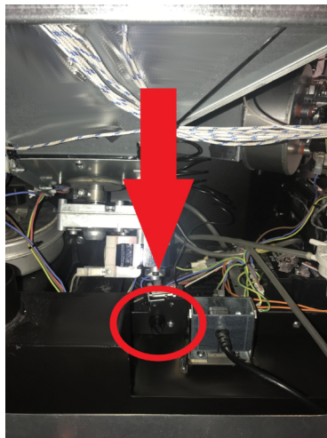
Fig. 40 - Riarmo manuale: si trova dietro al serbatoio, vicino alla spina di alimentazione
