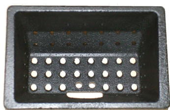
Fig. 28 - Voorbeeld van een schone brazier
