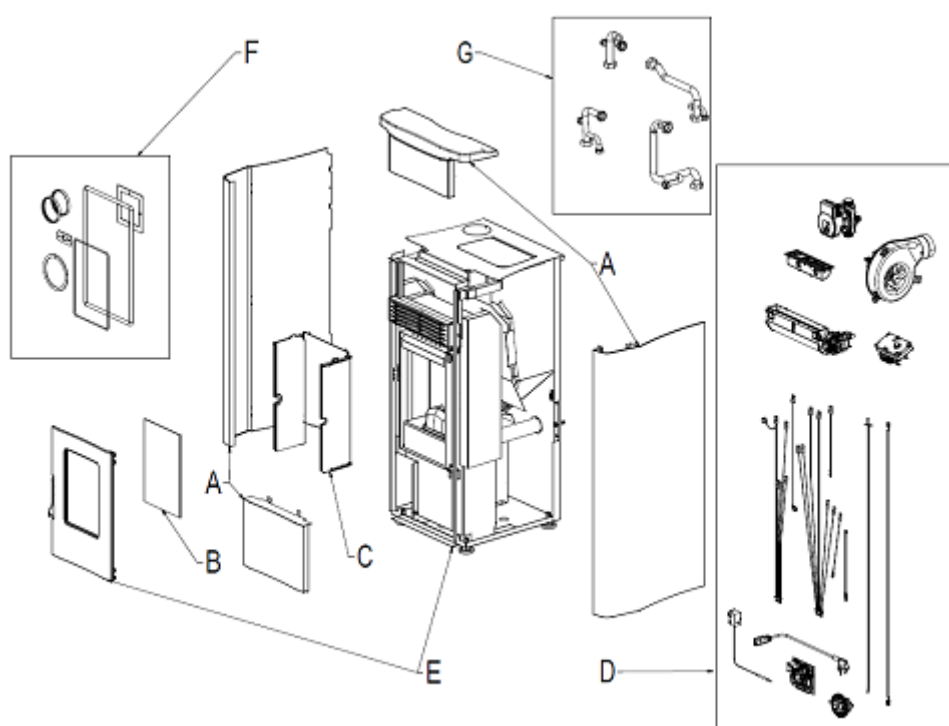
Fig. 1 - Dessin éclaté
