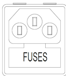
Fig. 35 - Hublot avec les fusibles à enlever
