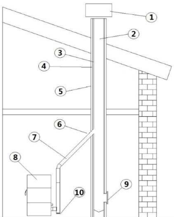
Fig. 2 - Componenti camino
