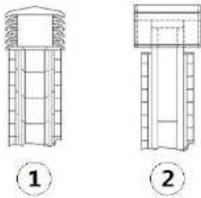
Fig. 5 - Comignoli antivento
