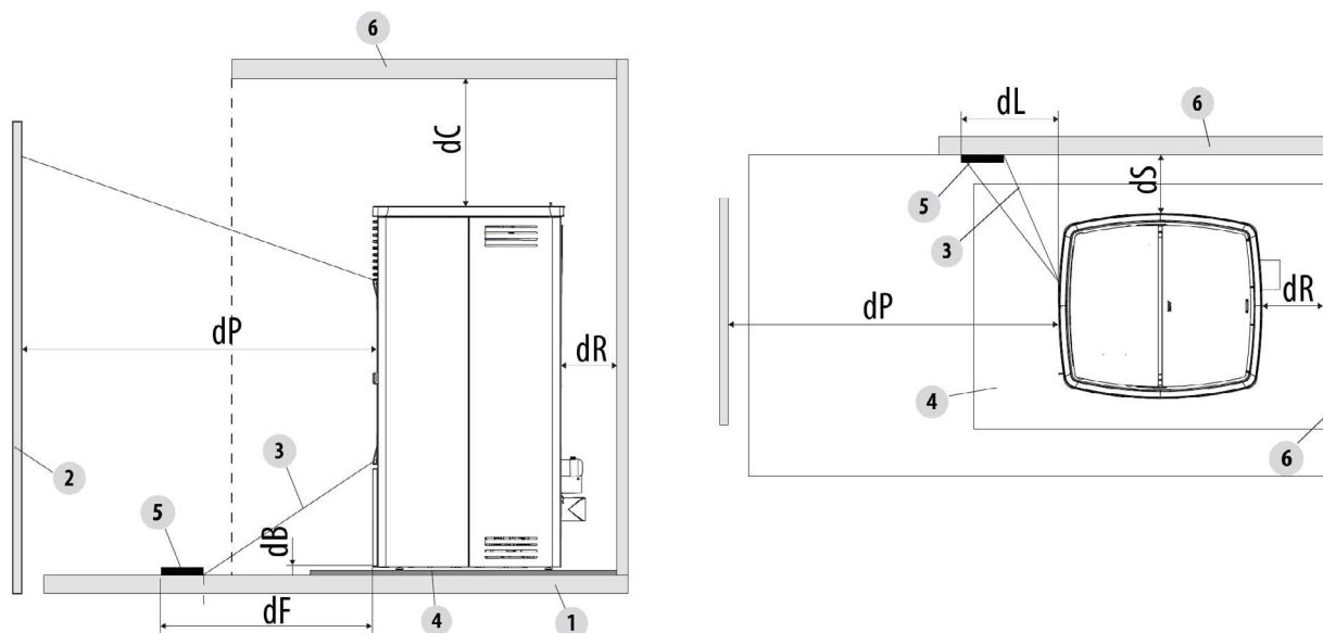
Fig. 11 - Distanze di sicurezza da materiale combustibile
