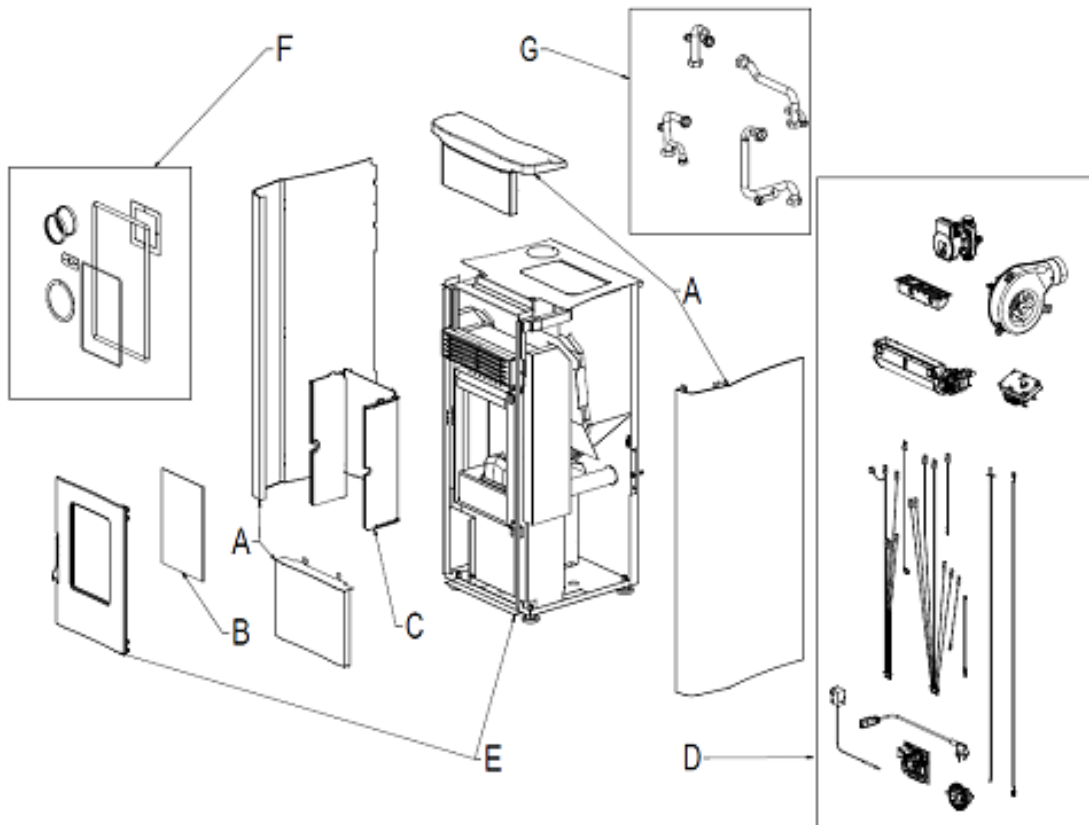
Fig. 1 - Esploso
