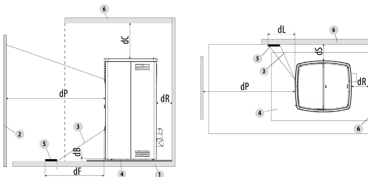
Fig. 9 - Sicherheitsabstand vom Brennstoff
