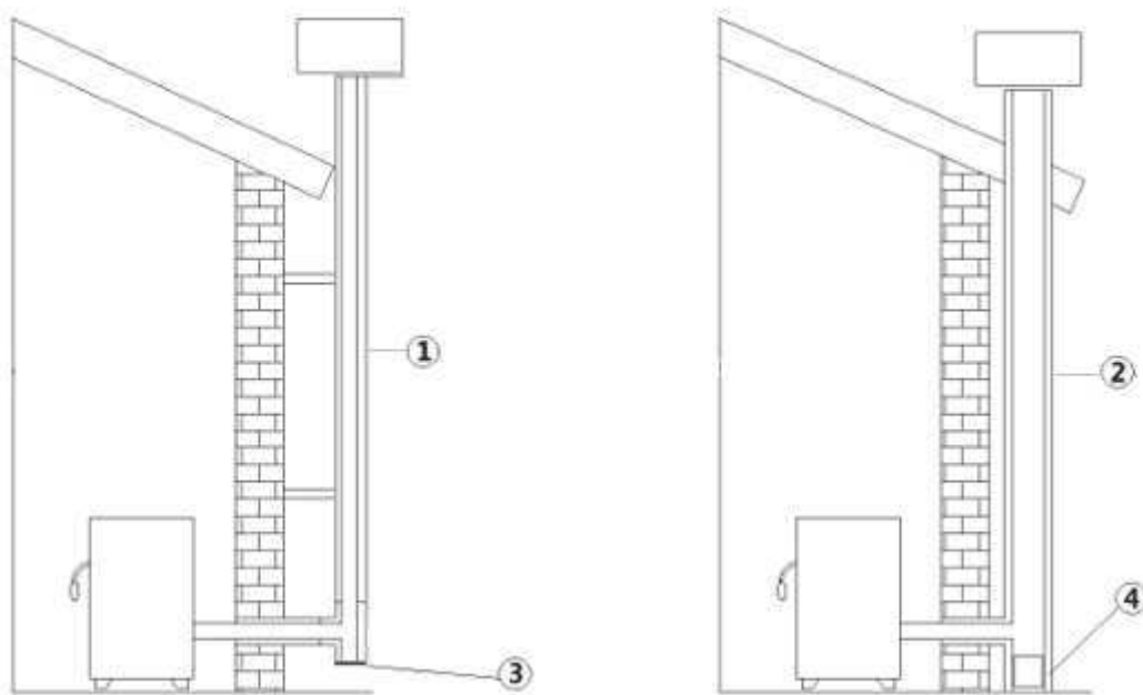
Fig. 3 - Rauchabzüge
