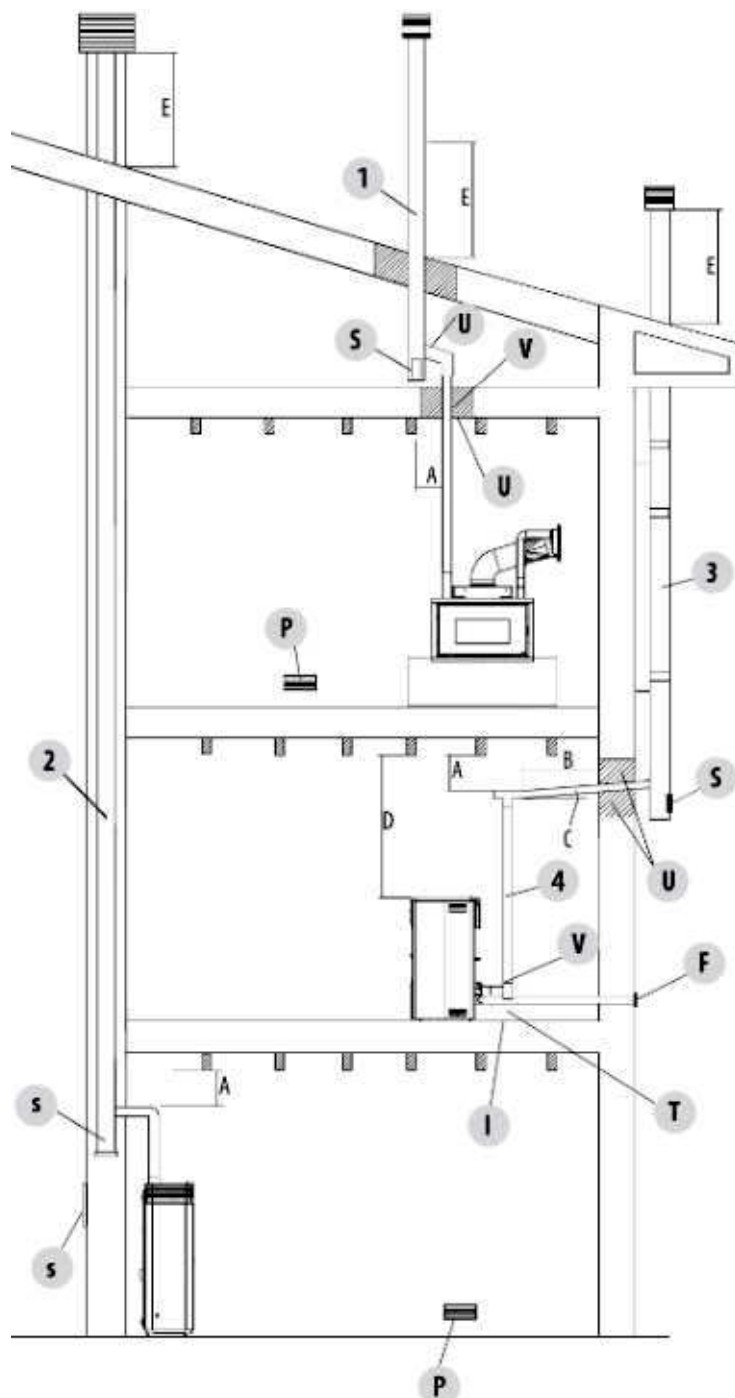
Fig. 8 - Rauchabzug
