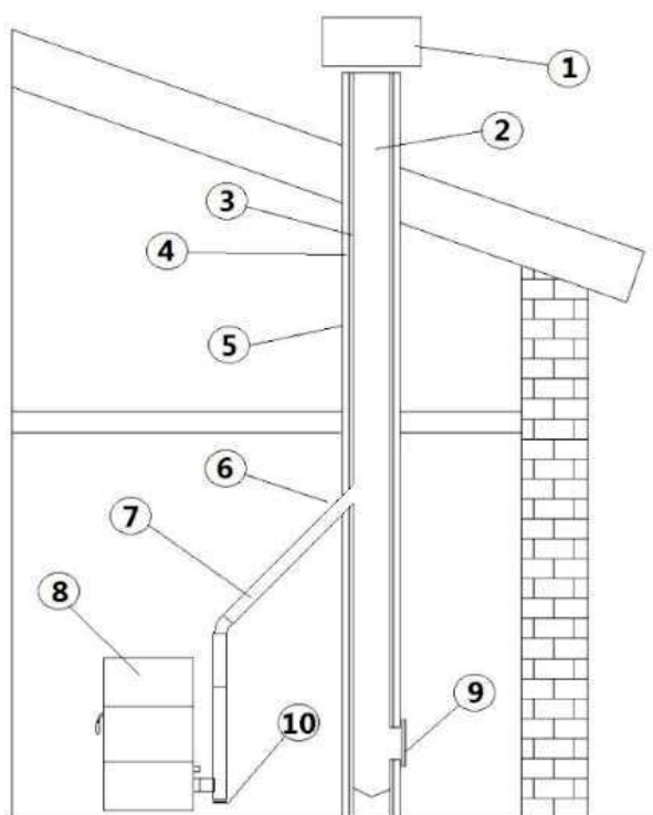
Fig. 2 - Bauteile Kamin
