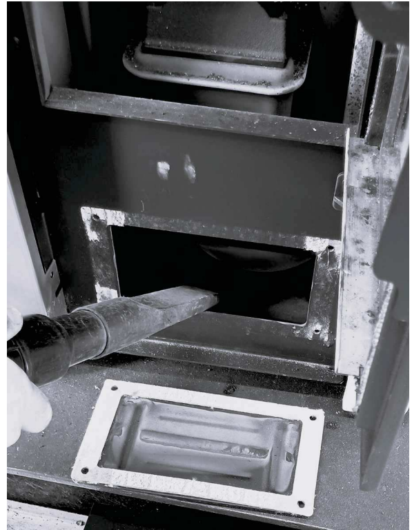
Fig. 29 - Die Asche absaugen
