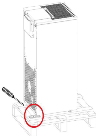
Fig. 1 - Entfernung der Halterungen
