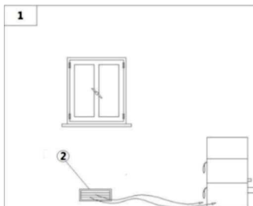
Fig. 7 - Direkte Luftzufuhr
