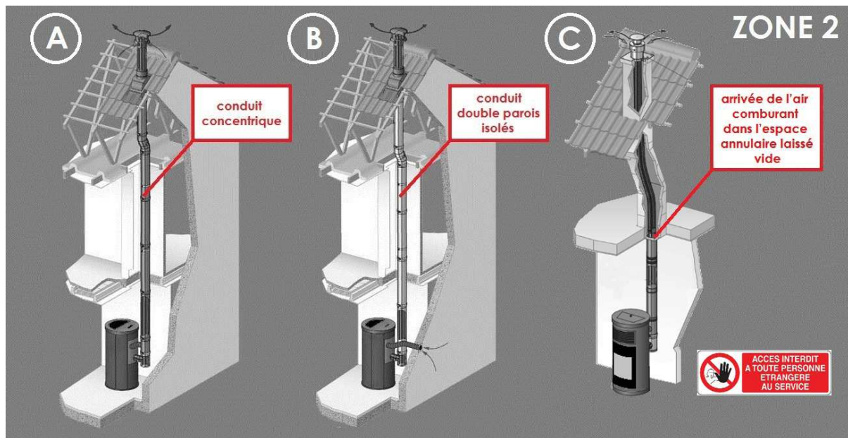
Fig. 14 - Schéma de principe des 3 types de système concentrique avec terminal vertical (ZONE 2)
