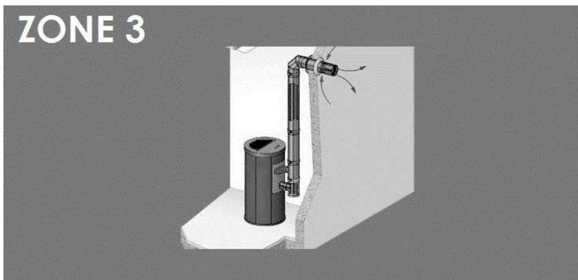
Fig. 15 - Schéma de principe du système concentrique avec terminal horizontal (ZONE 3)
