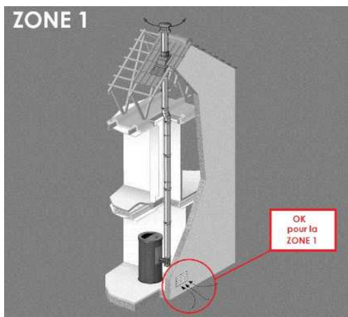
Fig. 13 - Installation possible pour tous les poêles (ZONE 1)
