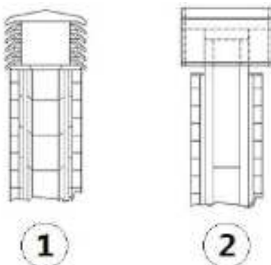
Fig. 6 - Sortie de toit coupe-vent
