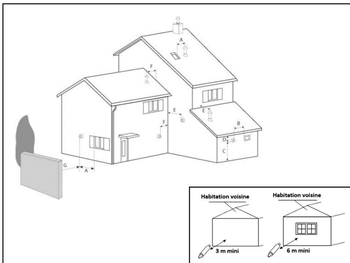
Fig. 11 - Position des terminaux
