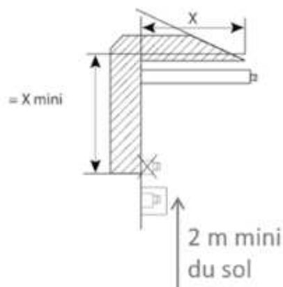
Fig. 12 - Rebord de toit
