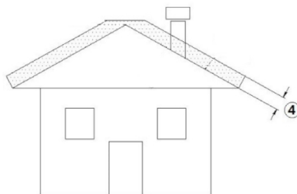
Fig. 5 - Refluxzone
