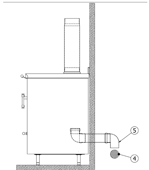
Fig. 7 - Indirecte luchttoevoer
