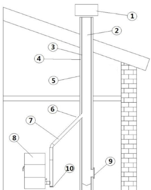
Fig. 2 - Onderdelen van de schoorsteen
