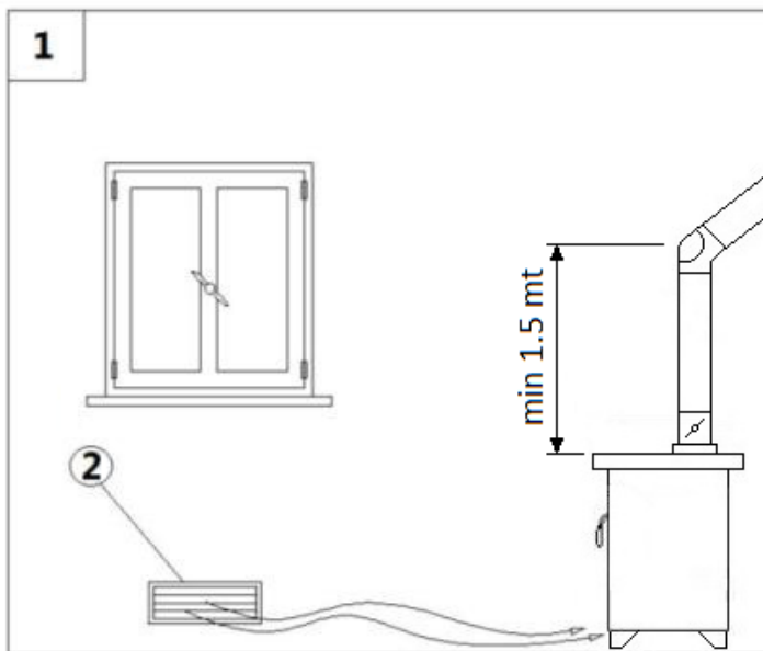
Fig. 6 - Directe luchttoevoer
