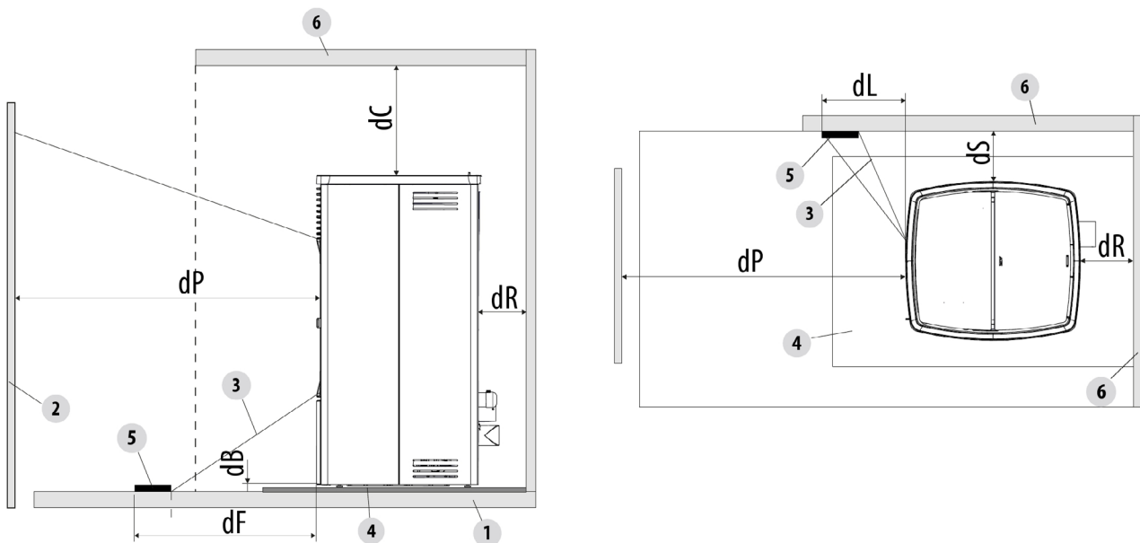
Fig. 11 - Veiligheidsafstand tot brandbaar materiaal (mm)
