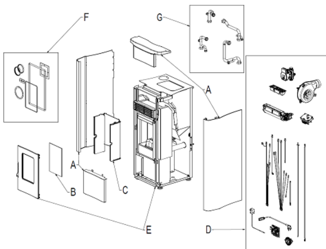
Fig. 1 - Dibujo explotado
