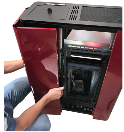
Fig. 55 - Entfernen der Platte
