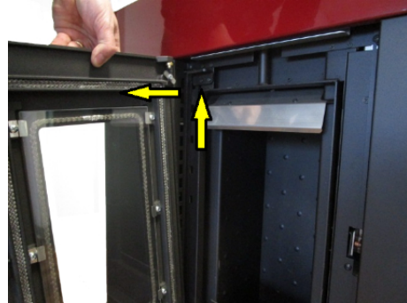
Fig. 27 - Ausbau der Tür
