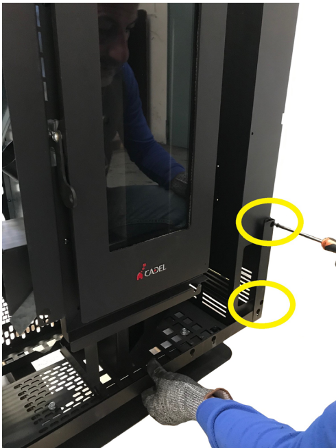
Fig. 34 - Befestigung des unteren Bügels
