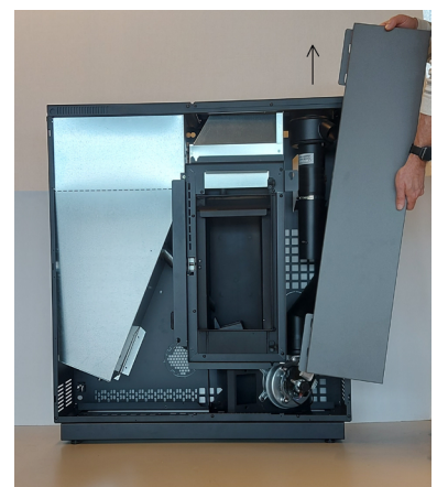
Fig. 66 - Demontage 6
