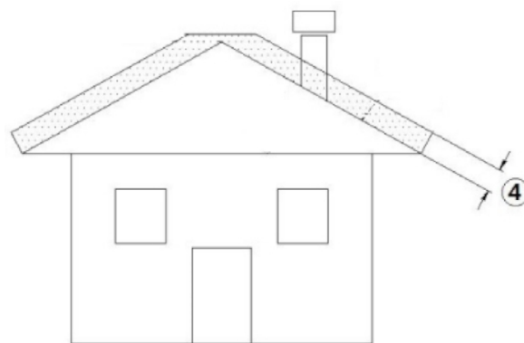
Fig. 6 - Rückflusszone
