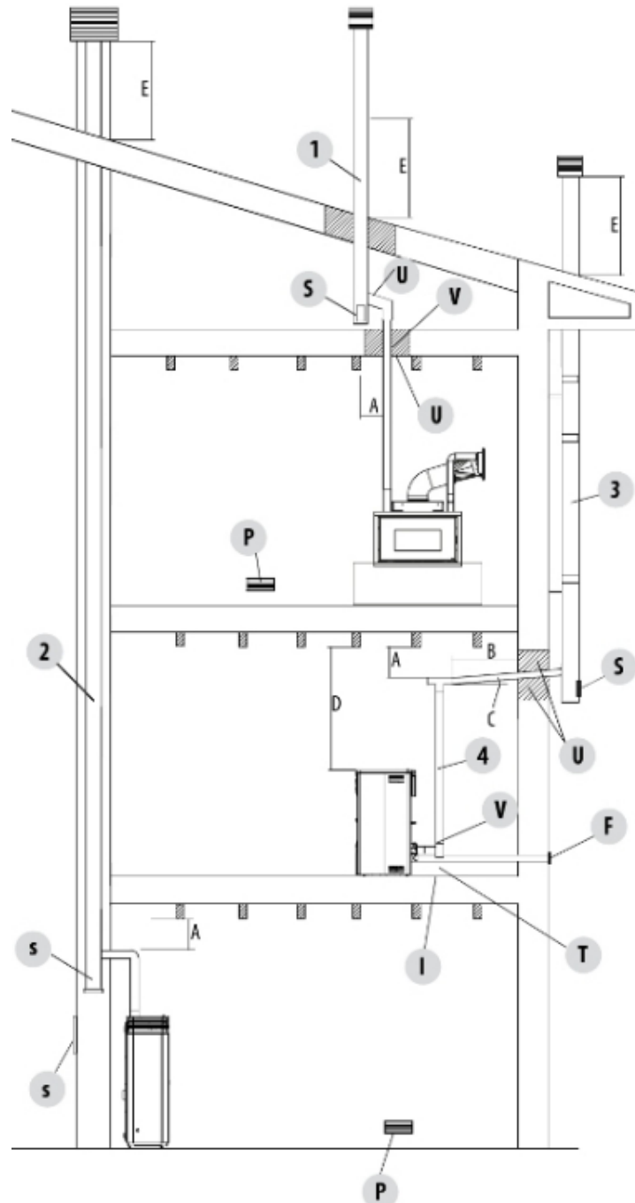
Fig. 10 - Rauchabzug
