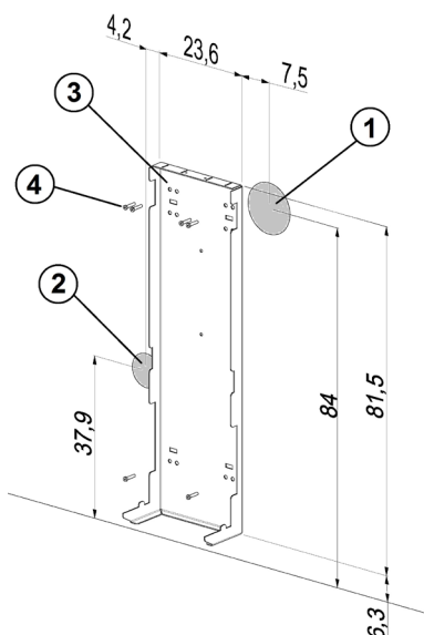
Fig. 79 - Step 1
