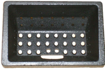
Fig. 32 - Beispiel einer sauberen Brennschale
