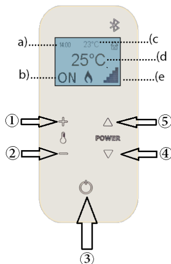
Fig. 31 - Fernsteuerung mit Thermostat
