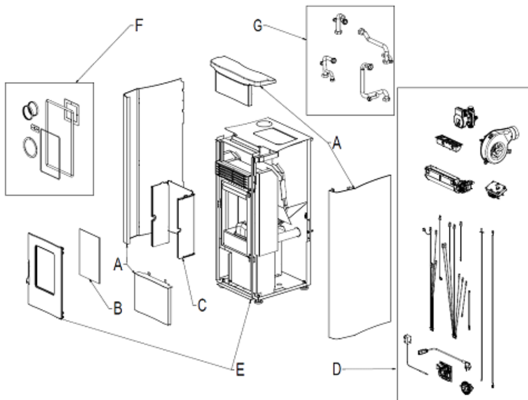
Fig. 1 - Explosionszeichnung
