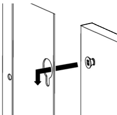
Fig. 55 - Détail de l'accrochage
