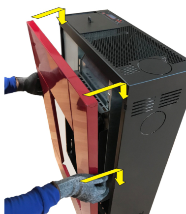
Fig. 41 - Fixation de l'encadrement au poêle
