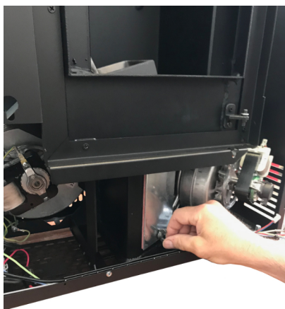
Fig. 97 - Retirer le bouchon d'inspection
