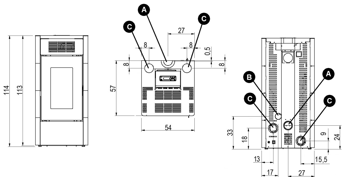
Fig. 14 - Dimensiones generales: Saba
