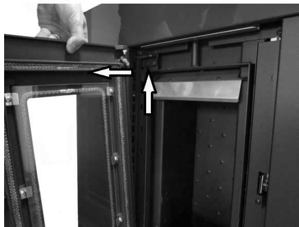
Fig. 16 - Desmontaje de la puerta
