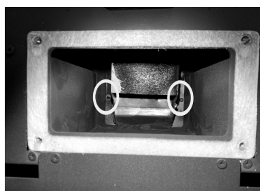
Fig. 65 - Desenrosque los tornillos
