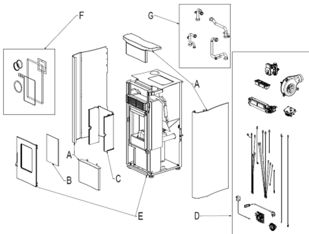
Fig. 1 - Explosionszeichnung
