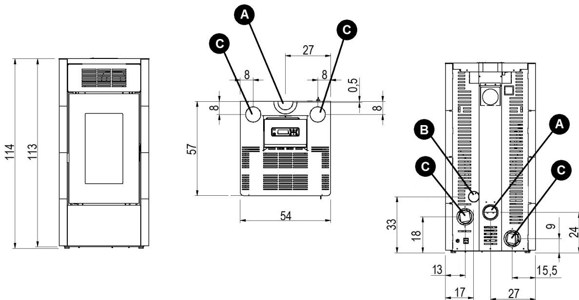
Fig. 21 - Dimensions générales: Saba
