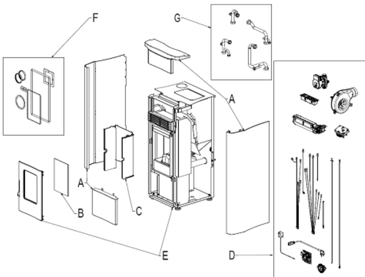
Fig. 1 - Dessin éclaté
