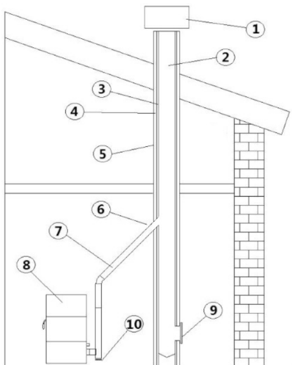
Fig. 2 - Componenti camino
