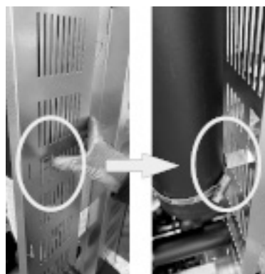
Fig. 37 - Piegare linguetta
