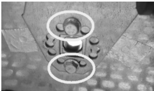
Fig. 69 - Rimozione viti
