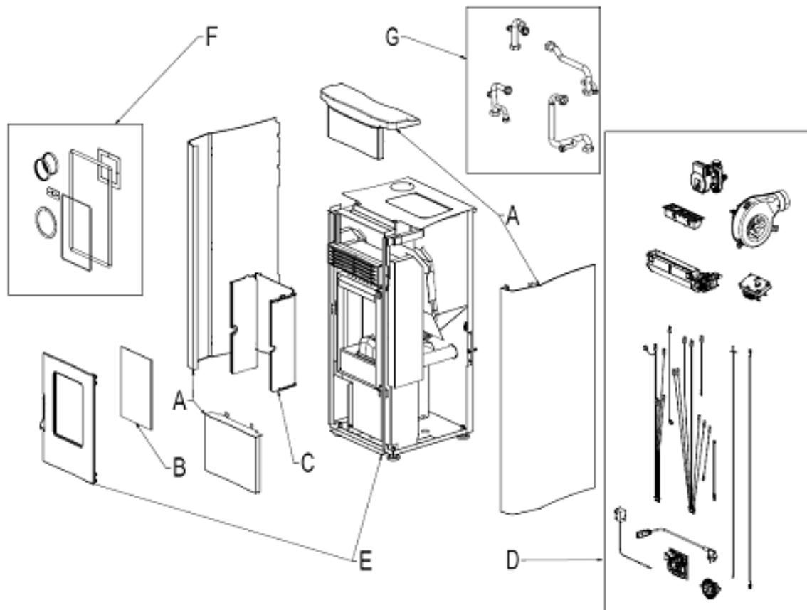
Fig. 1 - Explosionszeichnung
