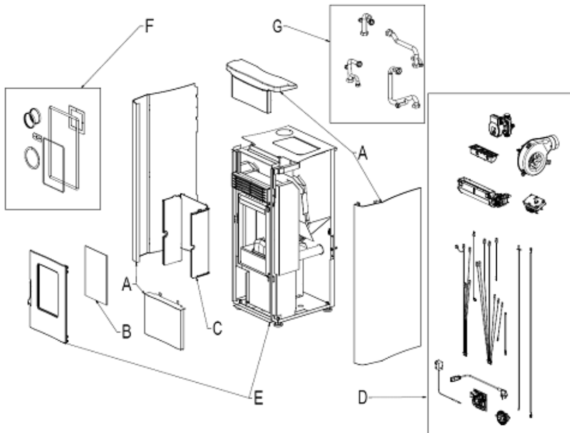
Fig. 1 - Dessin éclaté
