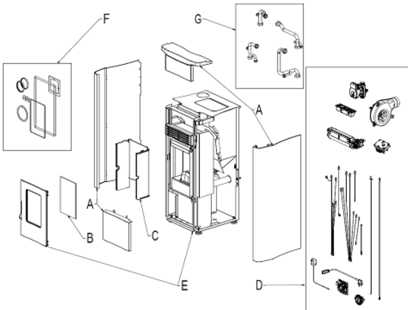
Fig. 1 - Esploso
