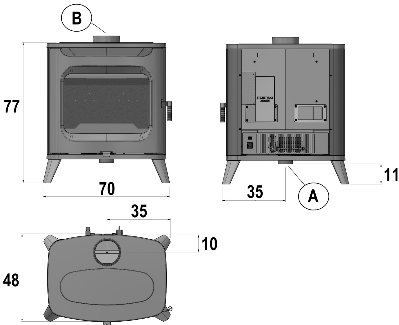
Fig. 11 - Dimensiones generales: HUBLLOT Wood
