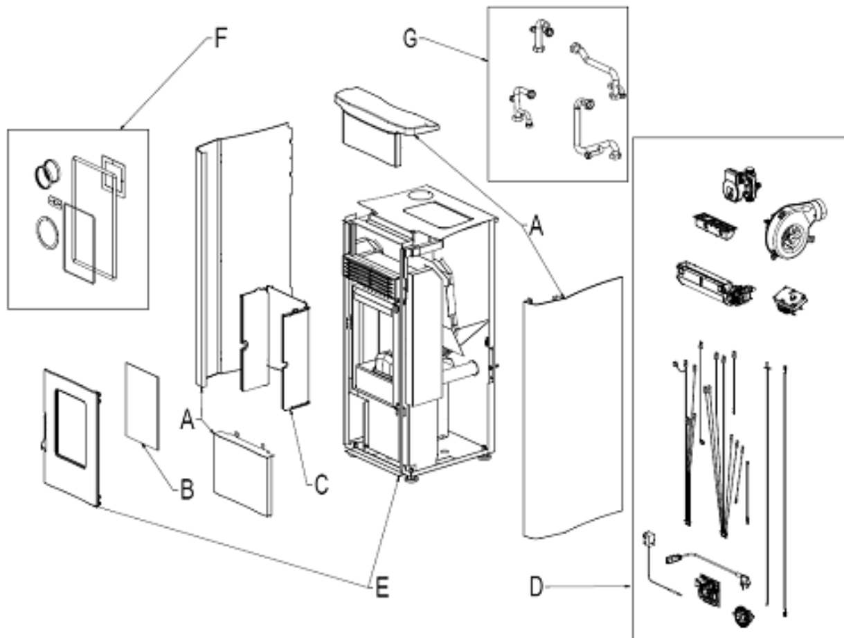
Fig. 1 - Dibujo explotado
