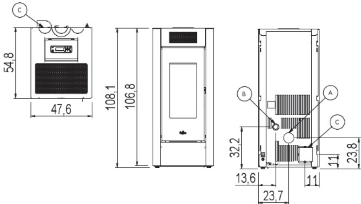
Fig. 14 - Dimensiones generales: Spark 11
