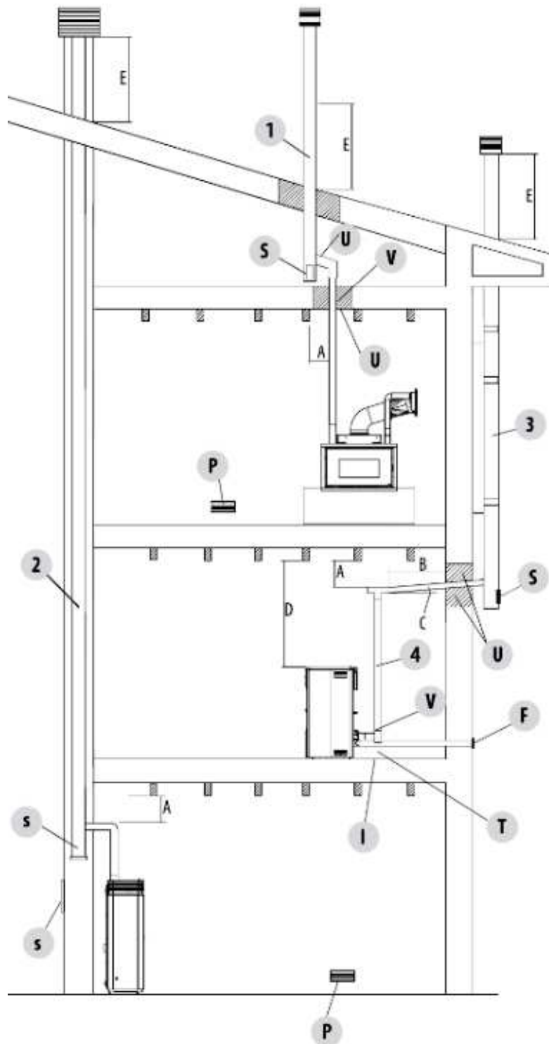
Fig. 12 - Sistema de evacuación de humos
