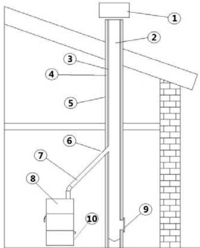
Fig. 2 - Componentes chimenea
