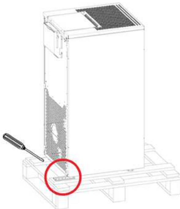
Fig. 1 - Extracción de las abrazaderas
