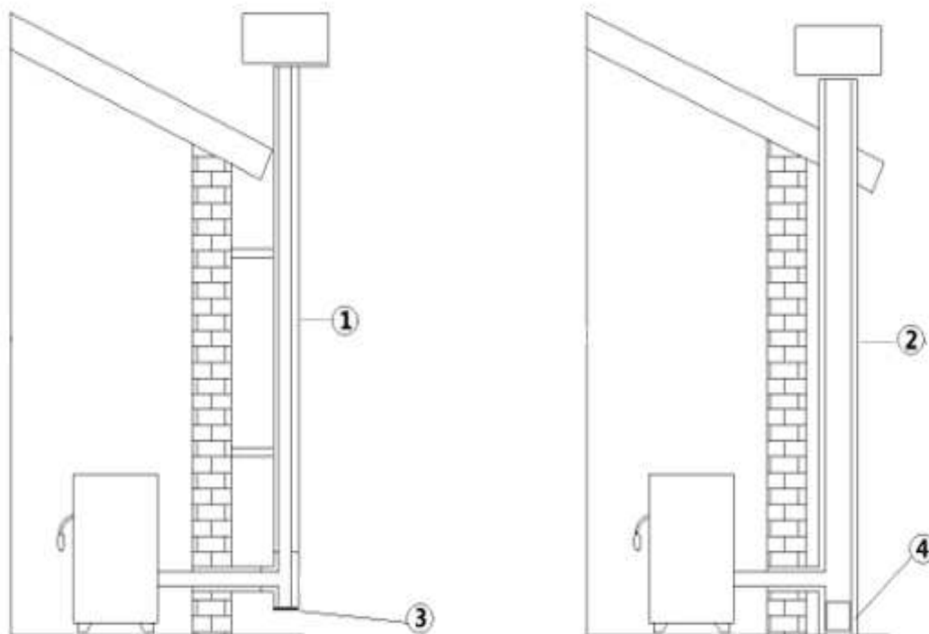
Fig. 5 - Conducto de chimenea
