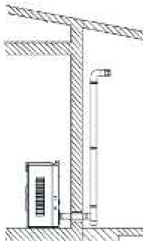
Fig. 4 - Salida "Ventouse" con codos y algunos metros de tubo más salida de techo (desaconsejado y prohibido)
