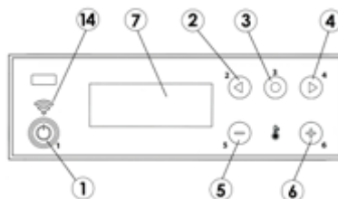
Fig. 6 - Panel de mandos (wi-fi)
