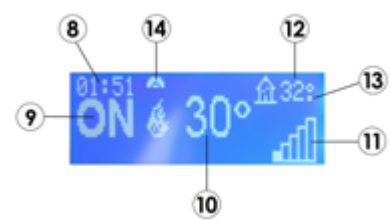
Fig. 7 - Display
