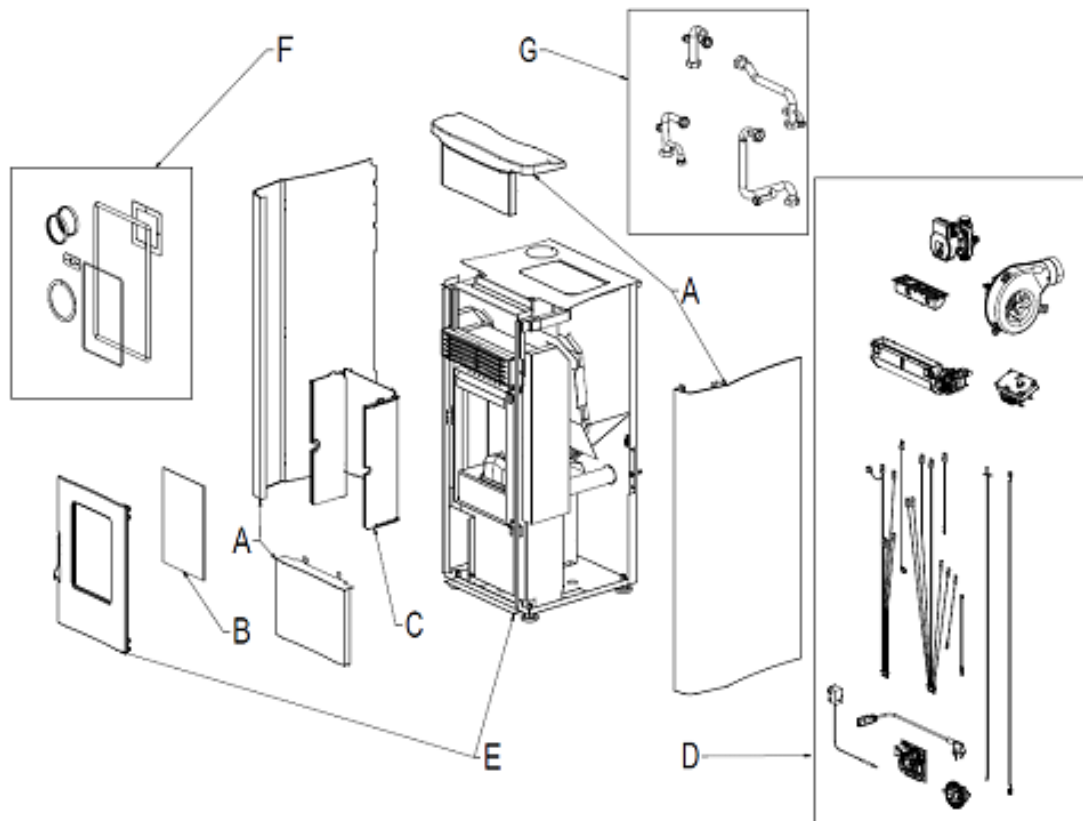
Fig. 1 - Dibujo explotado
