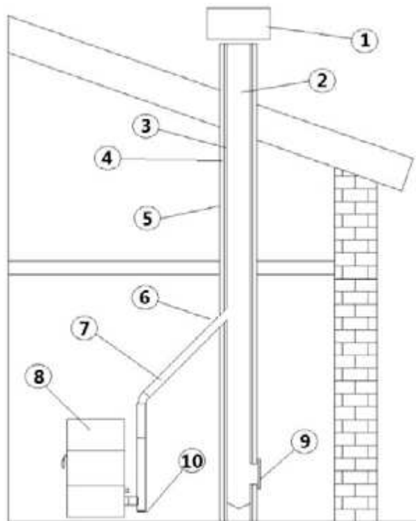
Fig. 2 - Bauteile Kamin
