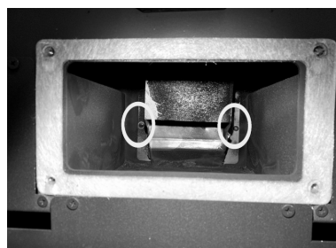
Fig. 63 - Die Schrauben lösen
