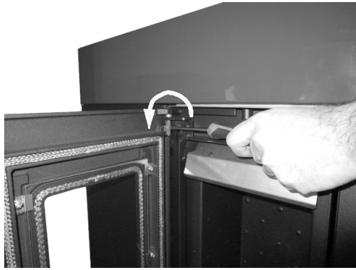
Fig. 13 - Entfernen der Schrauben
