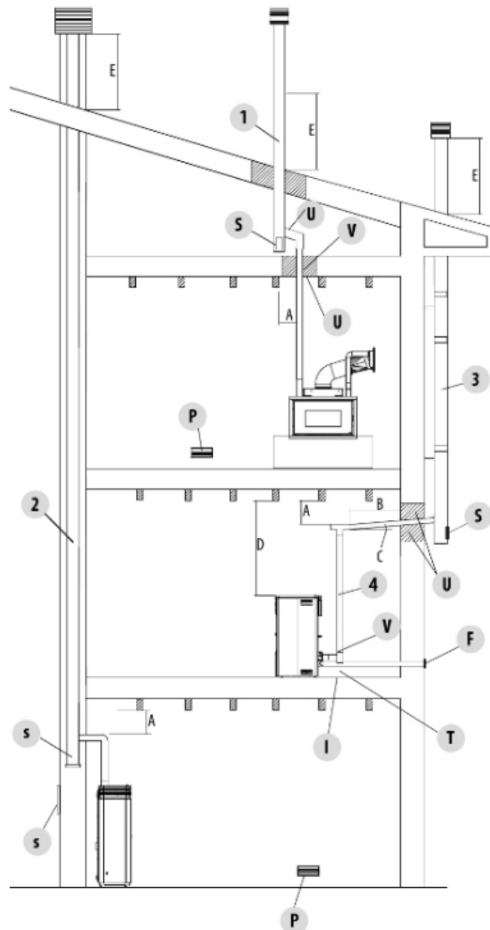
Fig. 10 - Rauchabzug
