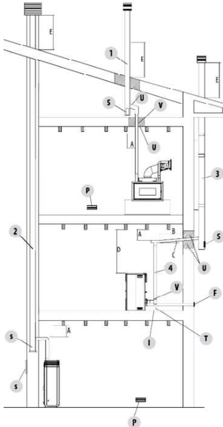
Fig. 10 - Rauchabzug
