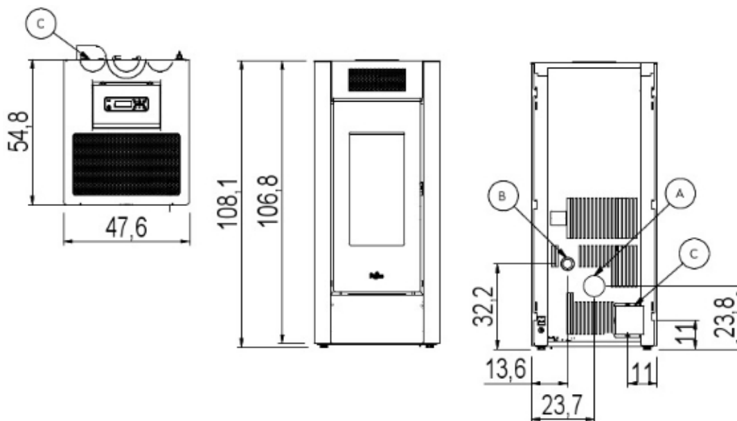
Fig. 12 - Allgemeine Abmessungen: Spark 11
