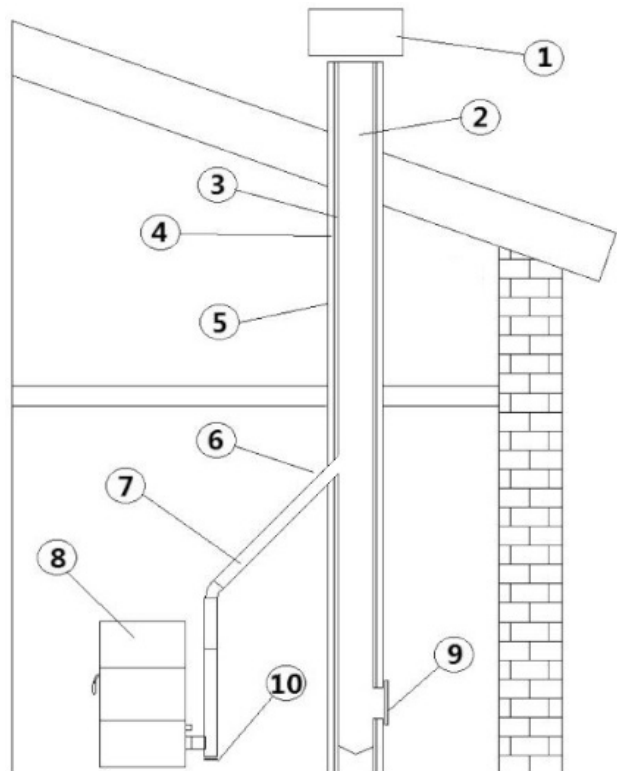
Fig. 2 - Bauteile Kamin
