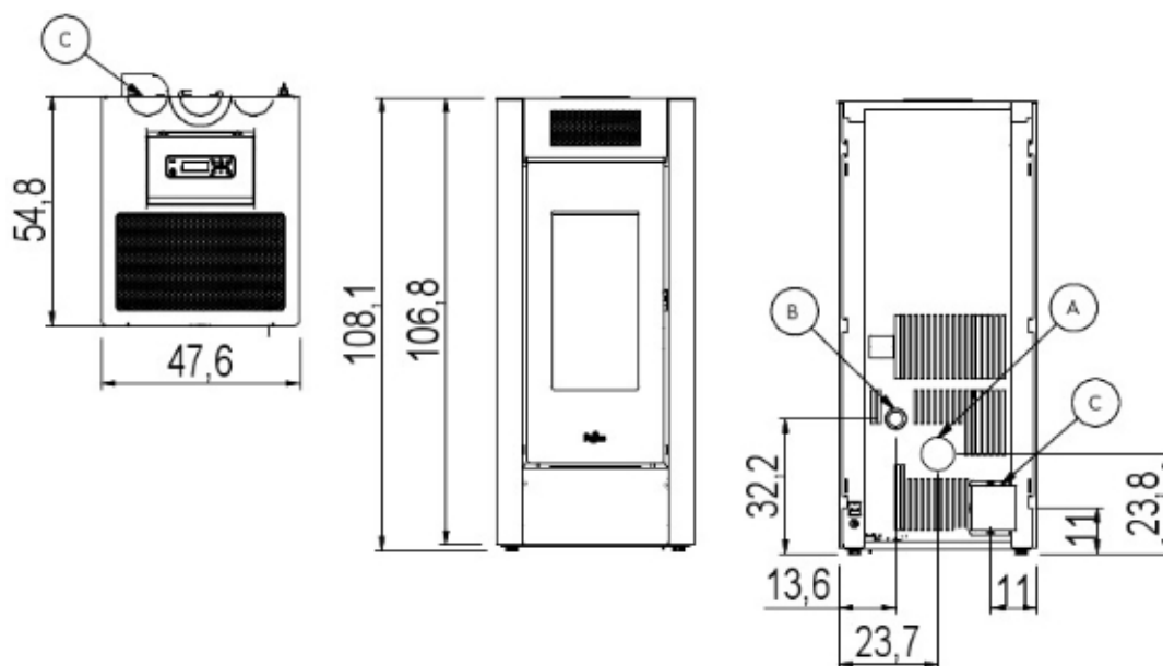
Fig. 21 - Dimensions générales: Spark 11
