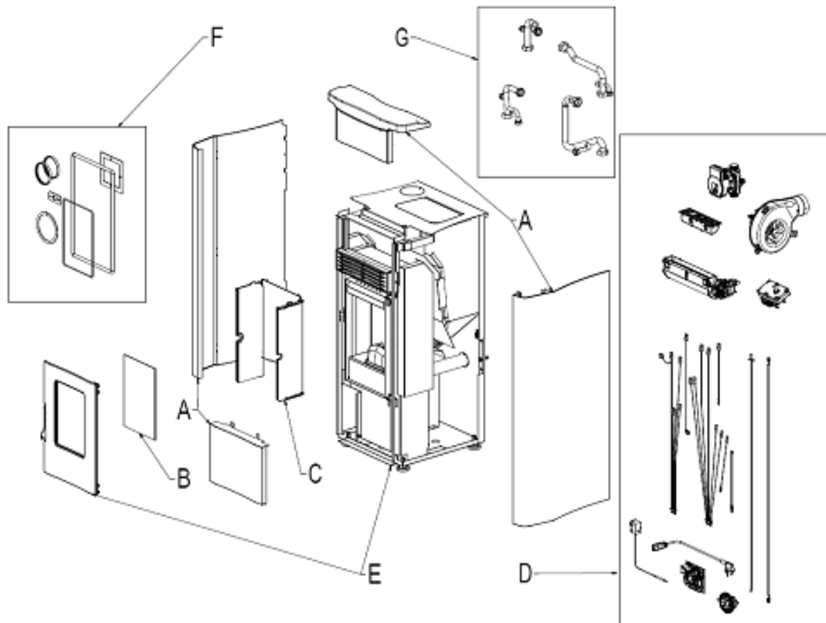
Fig. 1 - Dessin éclaté
