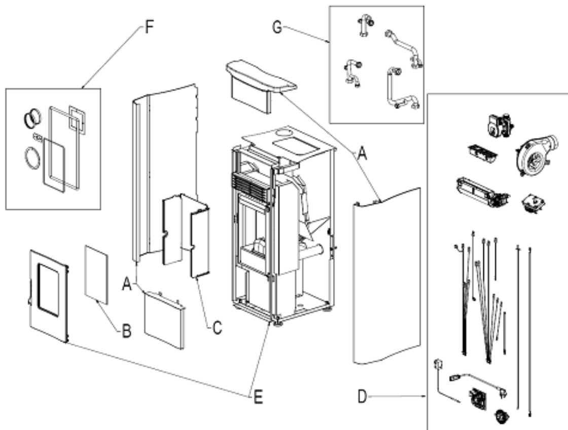
Fig. 1 - Esploso
