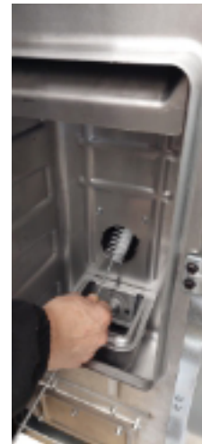
Fig. 43 - Reinigung mit Flaschenbürste
