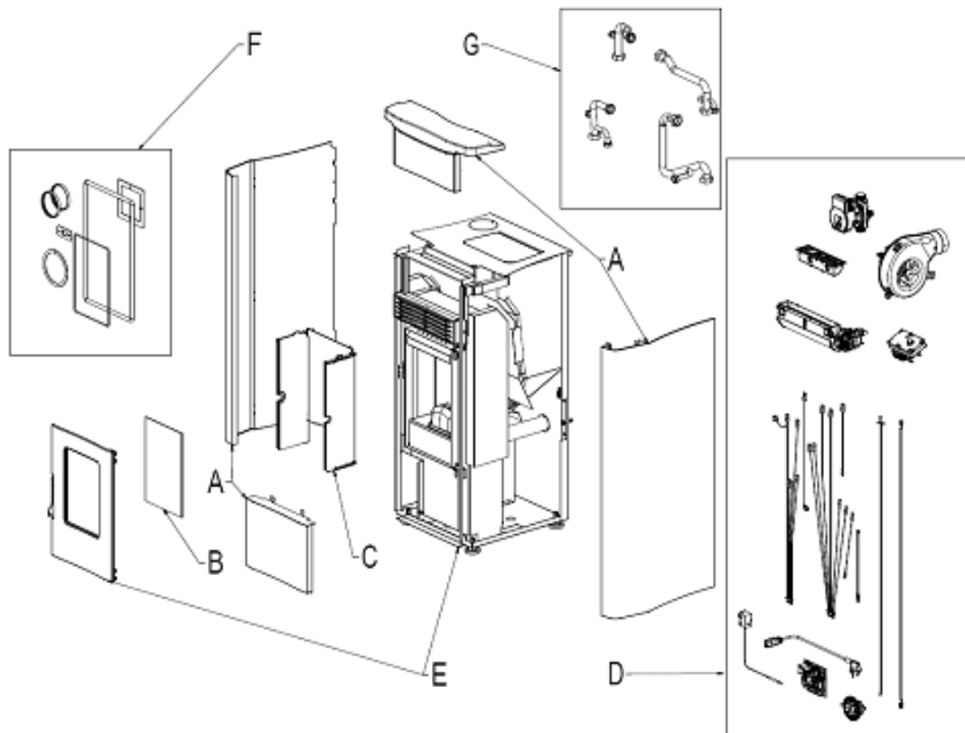
Fig. 1 - Dessin éclaté
