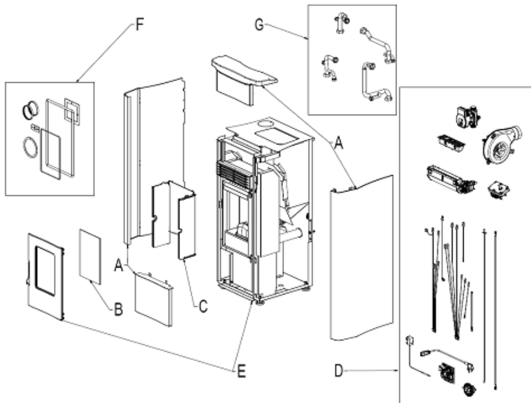
Fig. 1 - Explosionszeichnung
