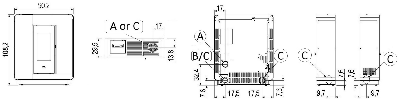
Fig. 23 - Elle Plus 7/9
