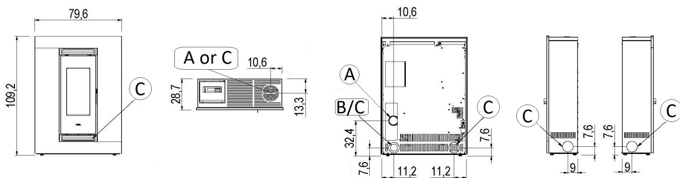
Fig. 21 - Luce Plus 7/9
