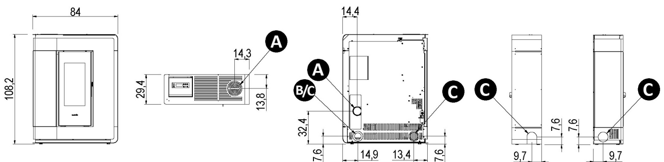
Fig. 25 - Arco 7/9
