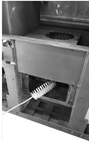
Fig. 71 - Nettoyer avec un goupillon
