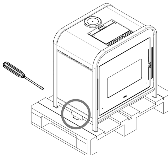
Fig. 1 - Lösen Schrauben + Biegel
