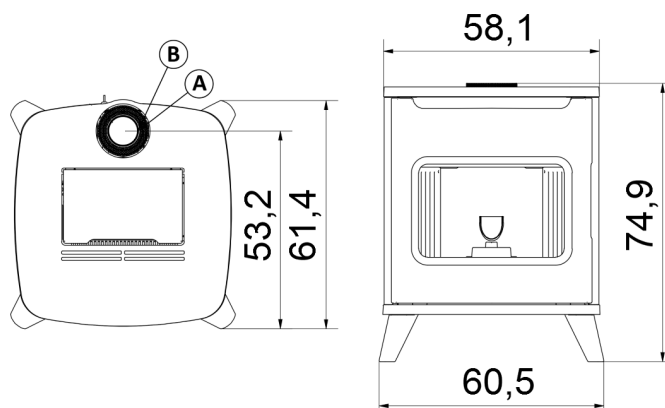
Fig. 13 - Dimensioni generali: HUBLLOT 6 UP
