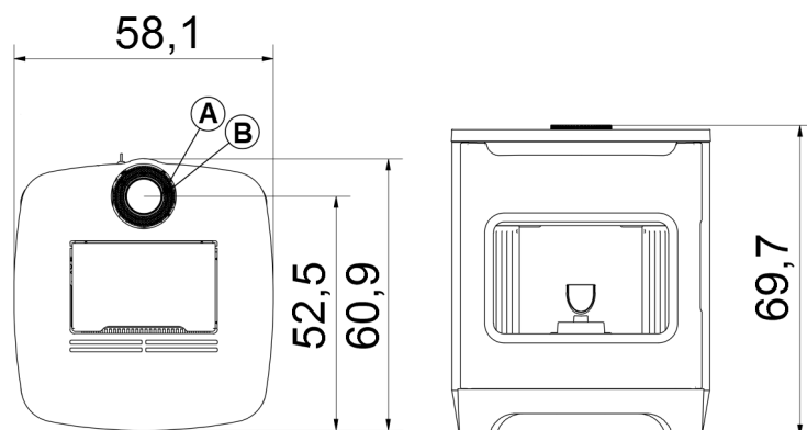
Fig. 14 - Allgemeine Abmessungen: FLOS 6
