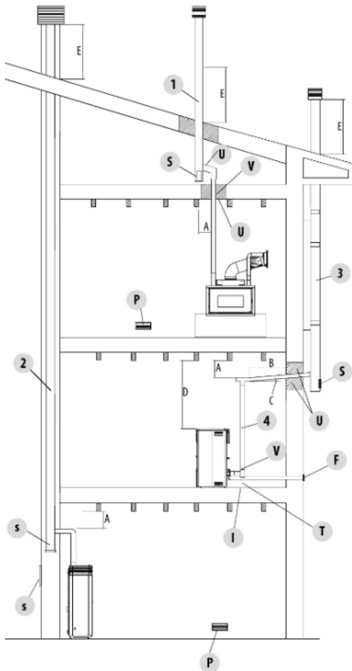
Fig. 10 - Rauchabzug
