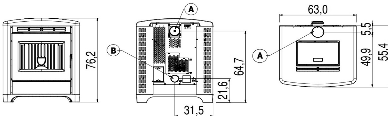
Fig. 12 - Allgemeine Abmessungen: MAGRITTE 6
