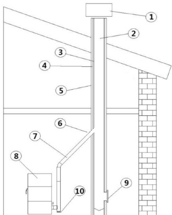
Fig. 2 - Bauteile Kamin
