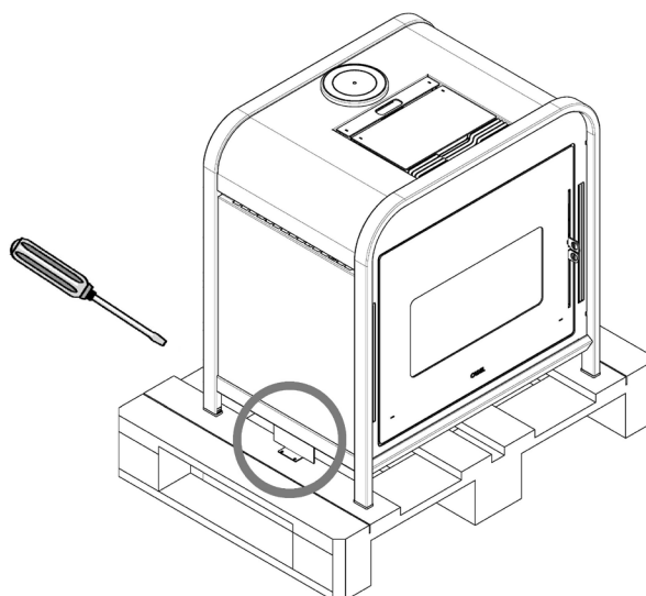
Fig. 1 - Retrait des vis + étriers
