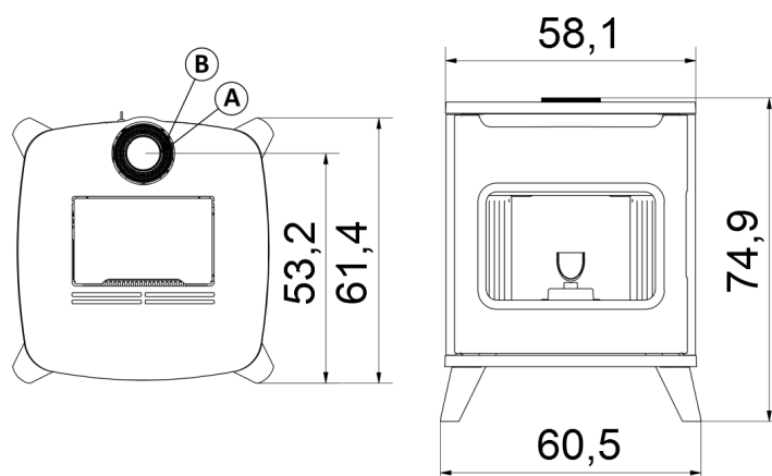
Fig. 22 - Dimensions générales: HUBLLOT 6 UP
