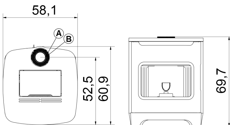
Fig. 23 - Dimensions générales: FLOS 6
