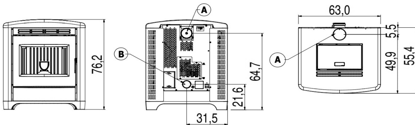
Fig. 21 - Dimensions générales: MAGRITTE 6
