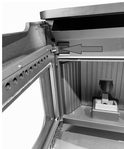
Fig. 26 - Réglage de la porte
