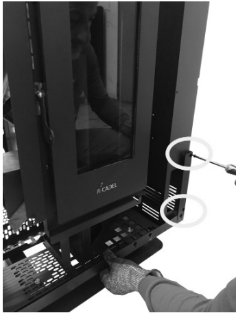
Fig. 33 - Befestigung des unteren Biegels
