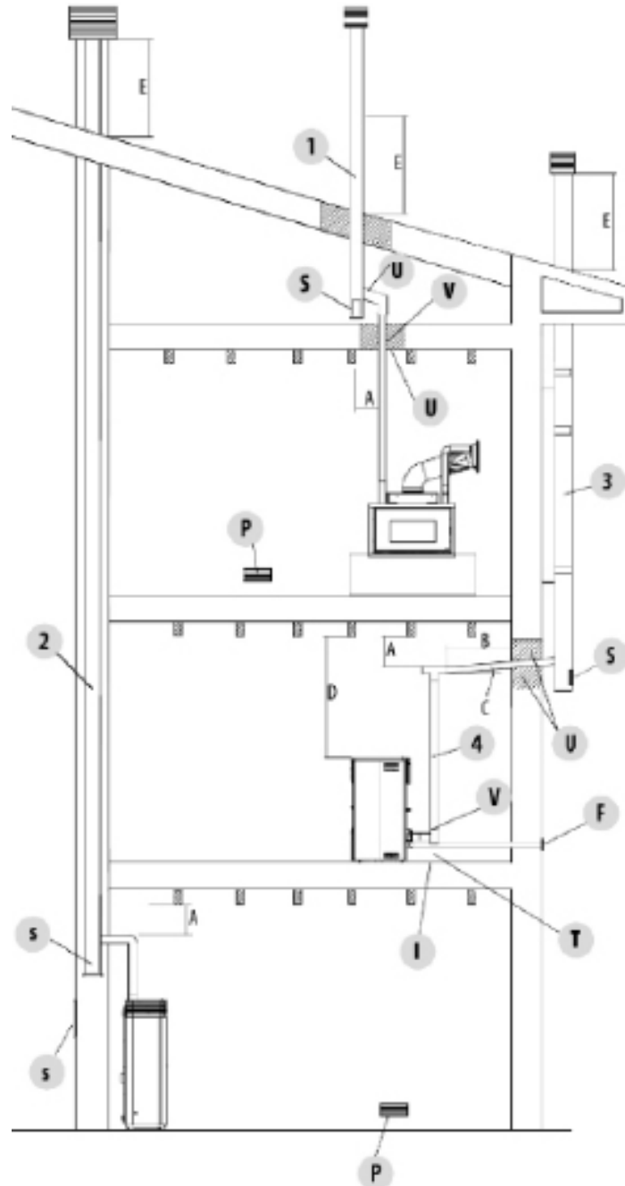
Fig. 10 - Rauchabzug
