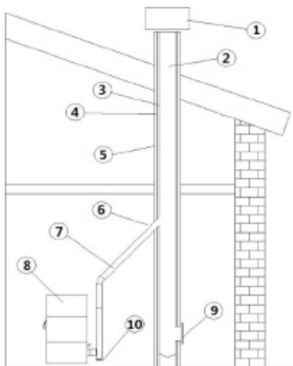
Fig. 2 - Bauteile Kamin
