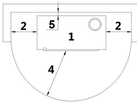
Fig. 57 - Wandinstallation
