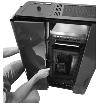
Fig. 47 - Entfernen der Platte
