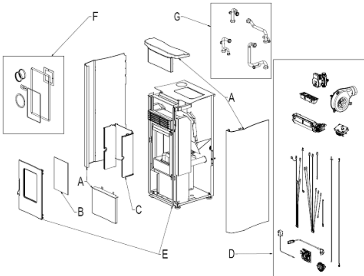
Fig. 1 - Dibujo explotado
