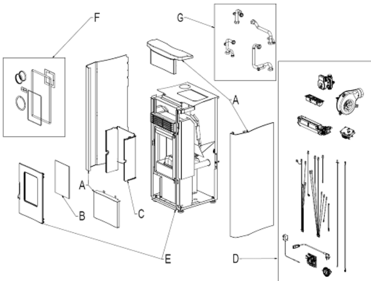
Fig. 1 - Esploso
