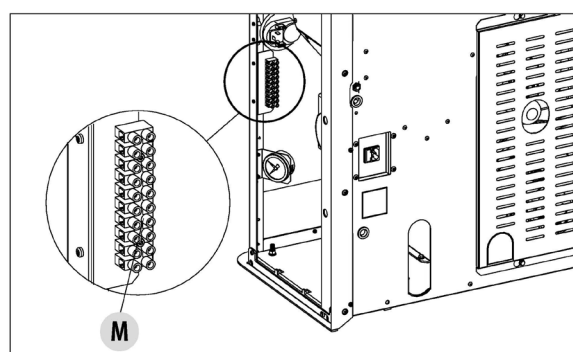
Fig. 75 - Collegamenti
