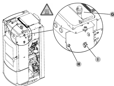
Fig. 63 - Valvola di sfiato manuale posta sotto il top (Idro Prince 3 16-23-23 H2O, Aquos 3 16-23-23 H2O, Idron 16-22 Airtight, Hidrofire 22.8)
