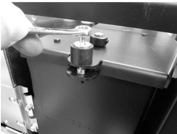
Fig. 91 - Svitare vite utilizzando chiave da 8
