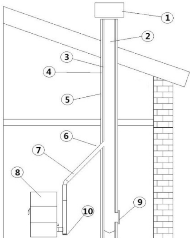
Fig. 5 - Componenti camino
