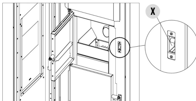
Fig. 79 - Chiusura sportello
