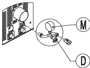
Fig. 62 - Terminale con rubinetto di caricamento (D) e manometro (M)
