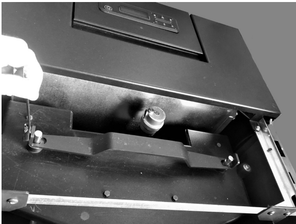
Fig. 89 - Svitare vite utilizzando chiave da 8
