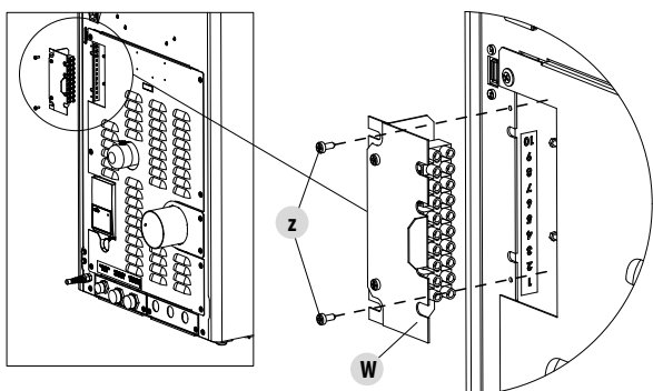
Fig. 74 - Collegamenti
