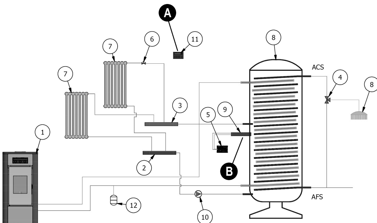
Fig. 70 - Configurazione 5
