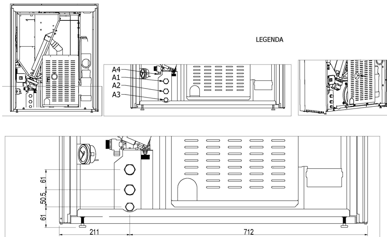
Fig. 60 - Schema allacciamento
