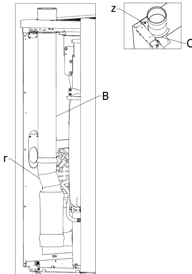
Fig. 57 - Uscita fumi superiore
