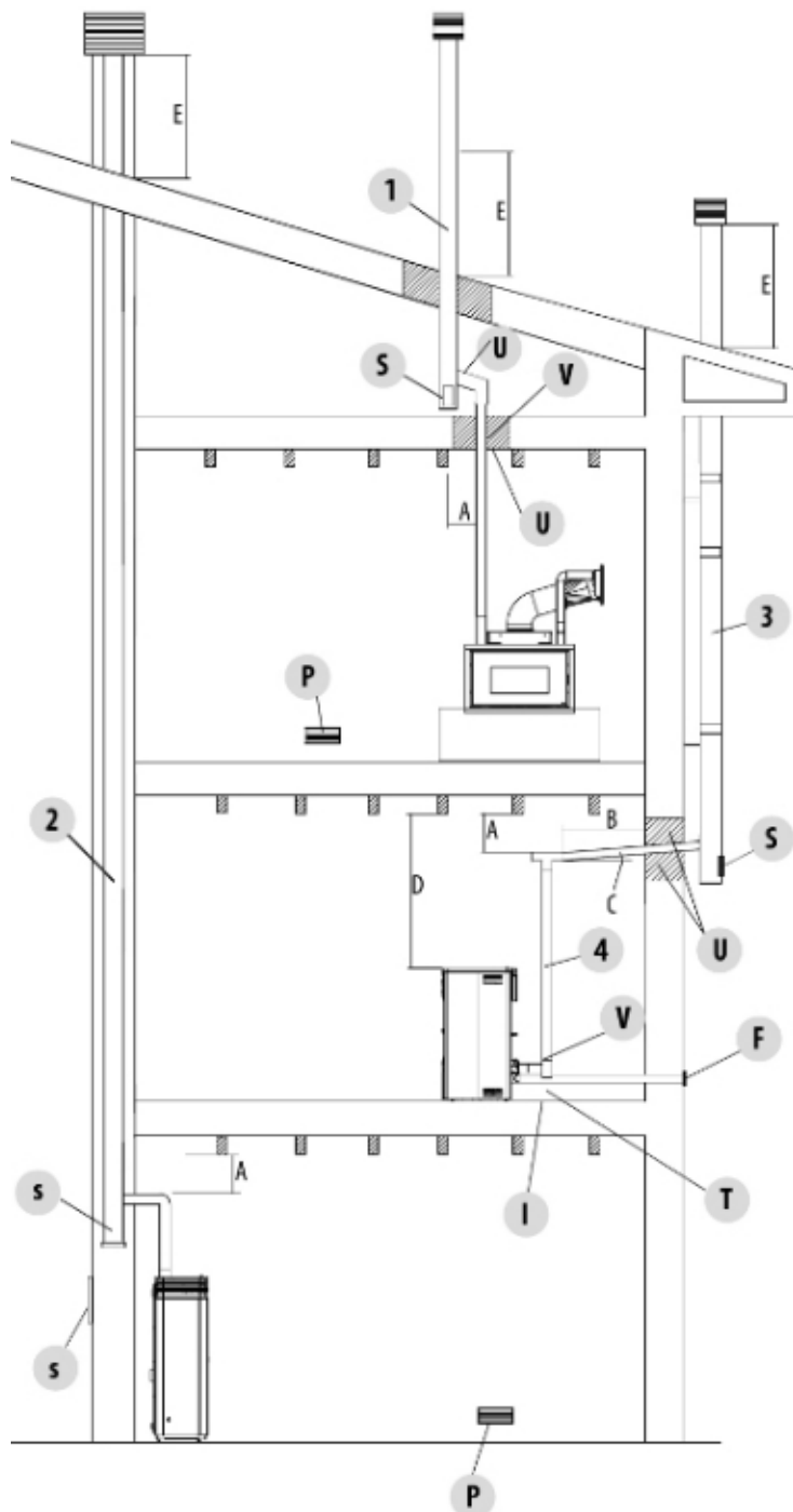
Fig. 13 - Canna fumaria
