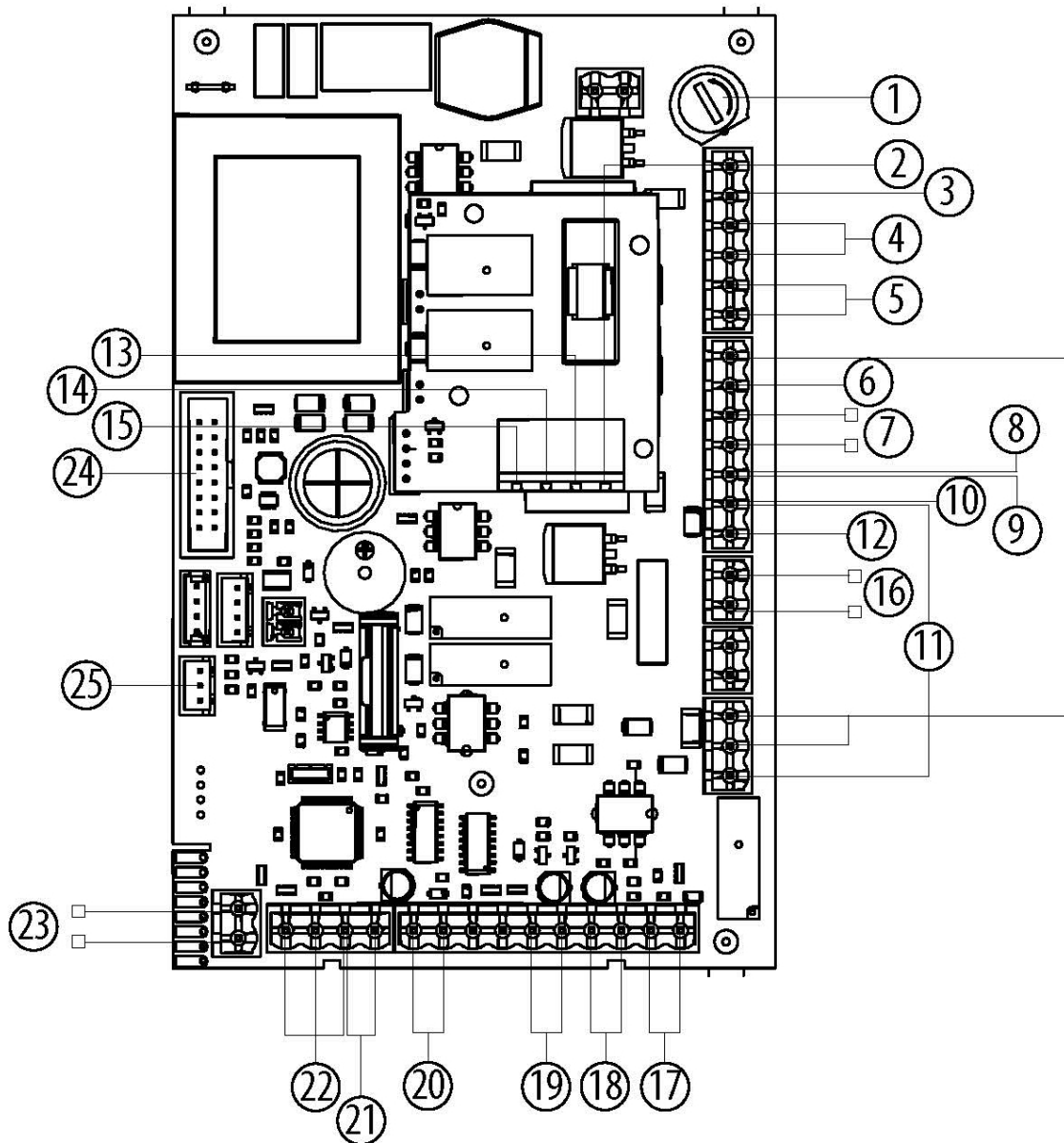
Fig. 99 - Scheda elettronica
