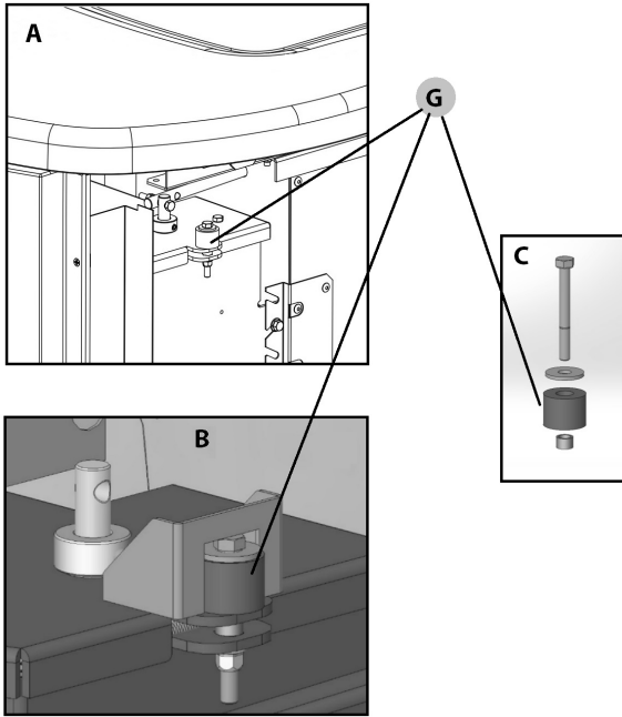
Fig. 87 - Gommino
