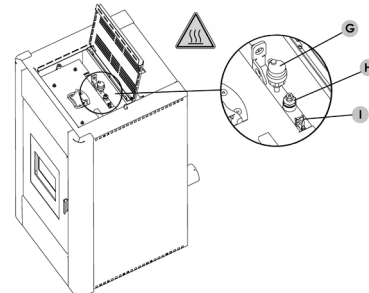
Fig. 64 - Valvola di sfiato manuale posta sotto il top (Idro Prince 3 30-30 H2O)
