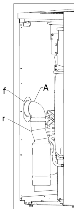
Fig. 56 - Uscita fumi posteriore
