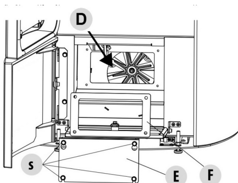
Fig. 78 - Pulizia vano inferiore
