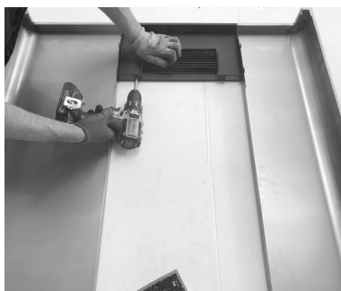
Fig. 39 - Fissaggio della griglia
