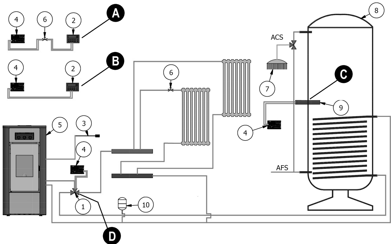
Fig. 68 - Configurazione 3
