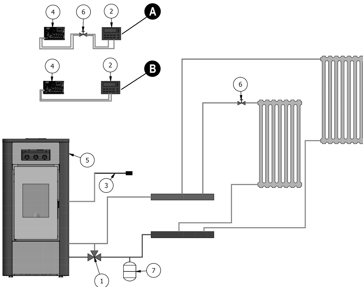
Fig. 65 - Configurazione 1
