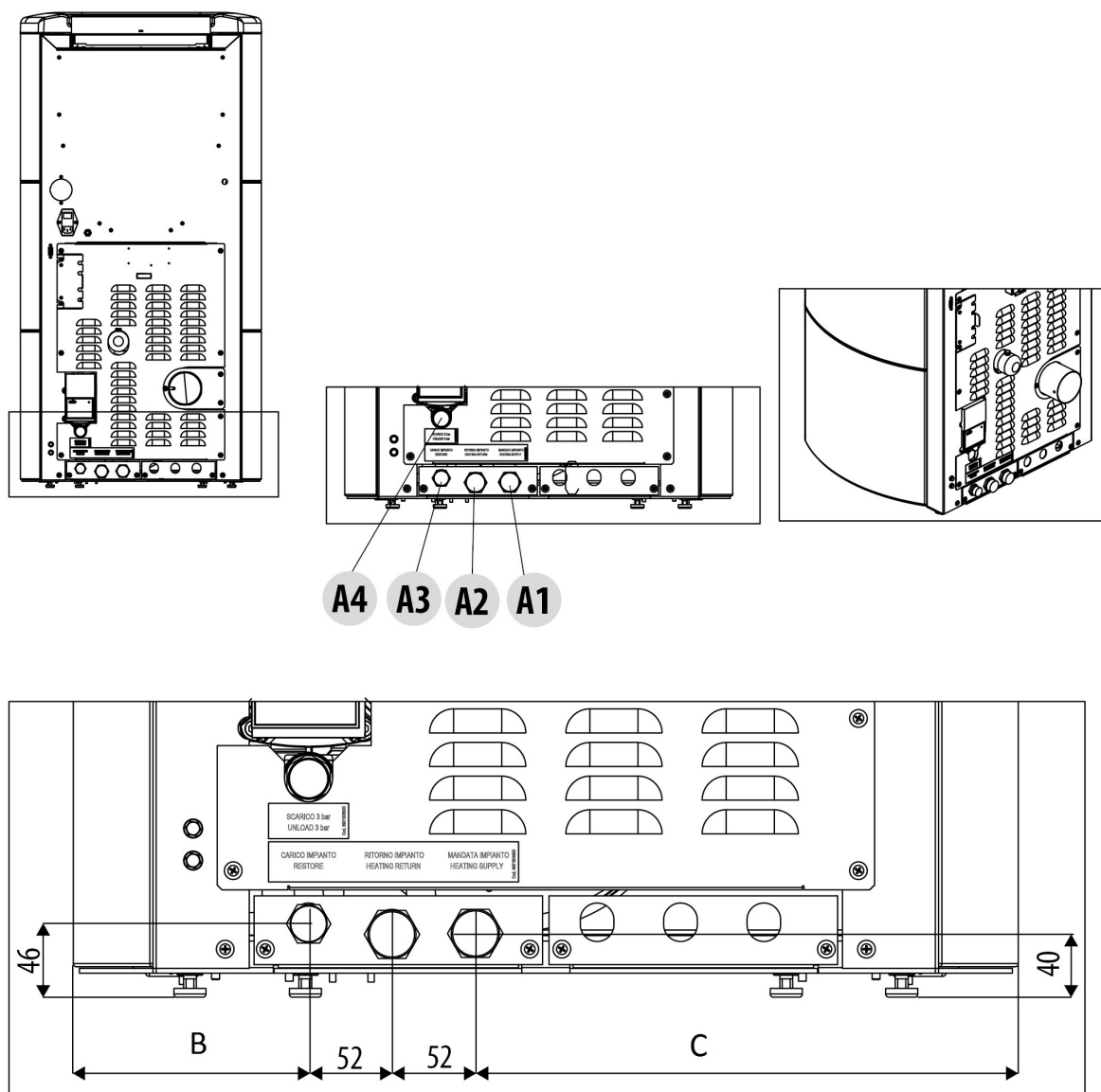
Fig. 58 - Schema allacciamento
