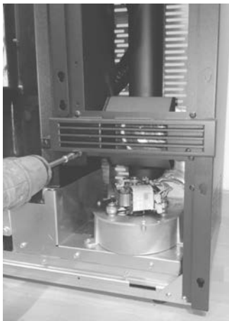
Fig. 56 - Bevestiging 1
