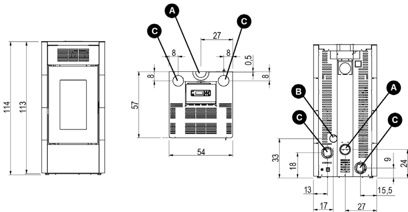
Fig. 14 - Algemene afmetingen: Saba 12/14
