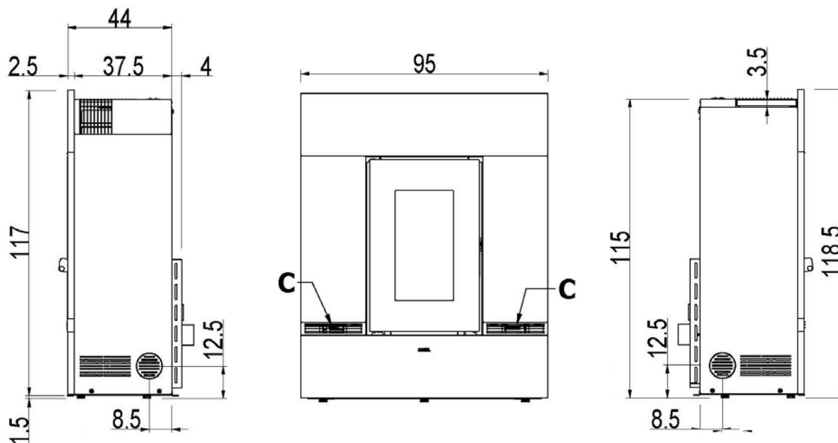
Fig. 17 - Algemene afmetingen: Mithos Plus 12/14 PS
