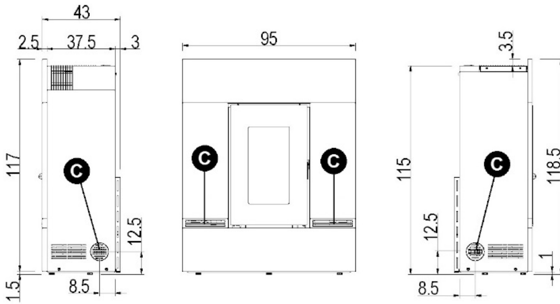
Fig. 15 - Algemene afmetingen: Mithos 3 Plus 12/14
