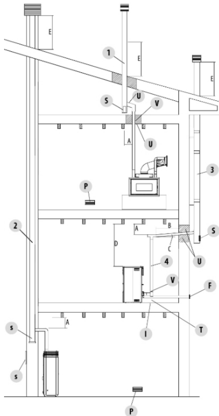
Fig. 10 - Rookkanaal
