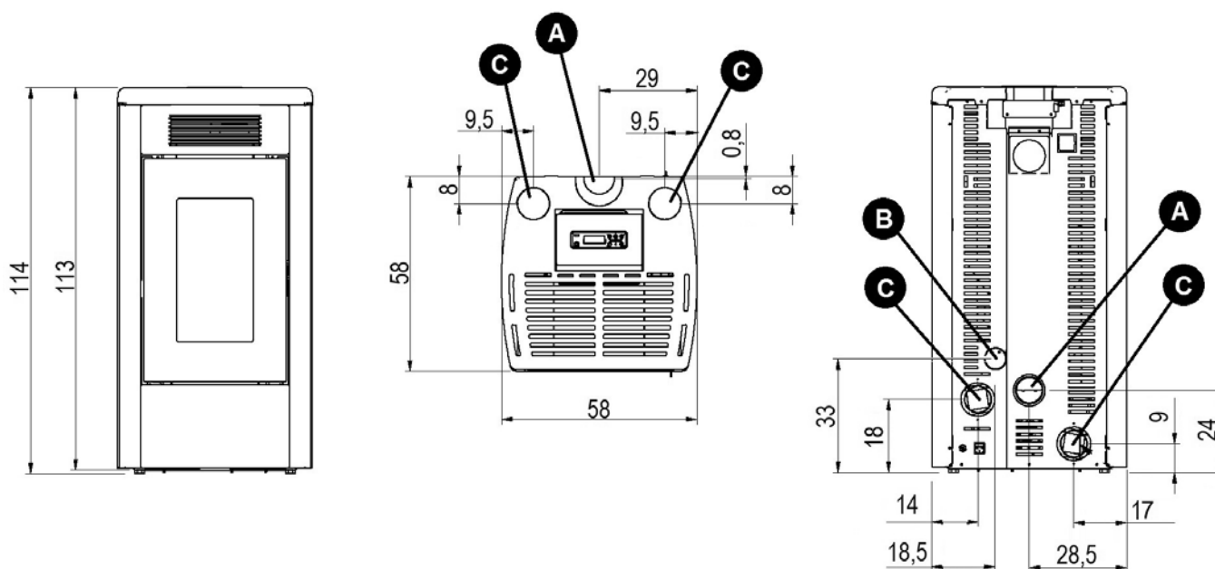
Fig. 12 - Algemene afmetingen: Atena 3 Plus 12/14
