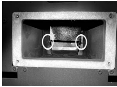
Fig. 125 - Draai de schroeven los
