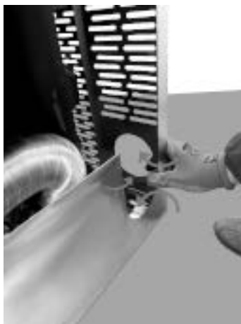
Fig. 88 - De tongetjes plooiën
