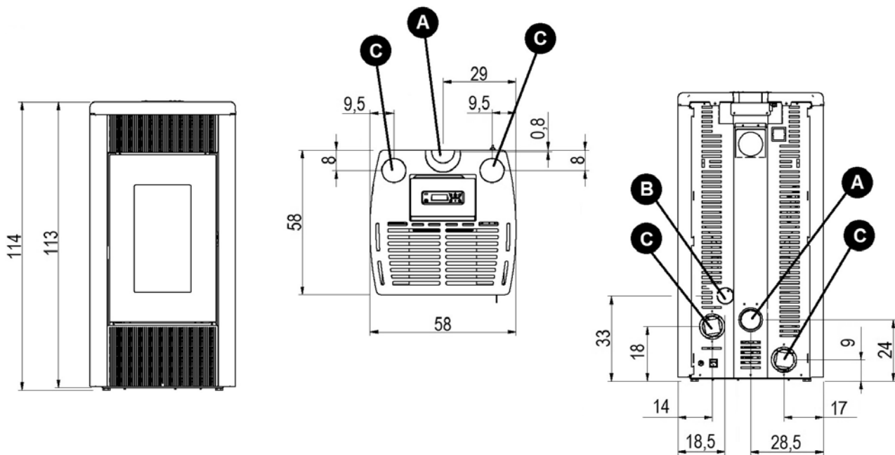
Fig. 13 - Algemene afmetingen: Duke 12/14 Airtight
