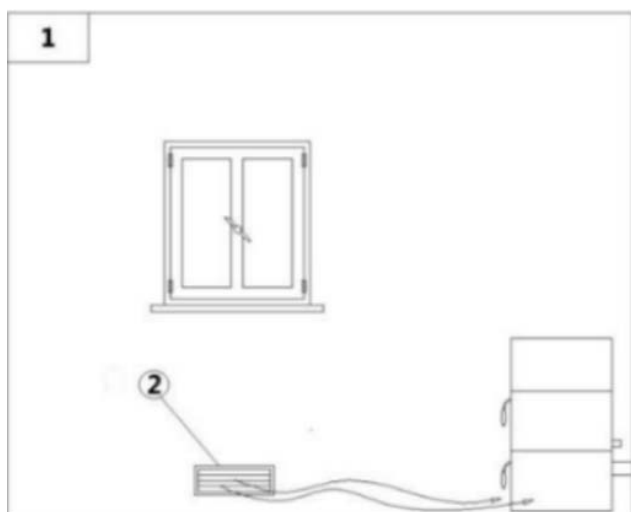
Fig. 7 - Directe luchttoevoer
