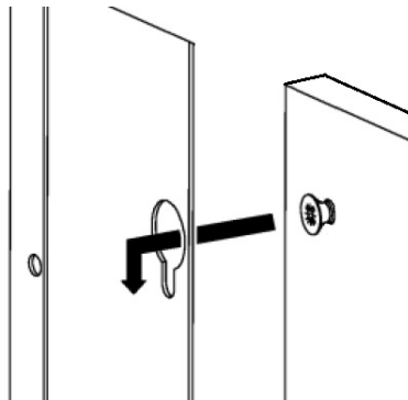
Fig. 61 - Detail van het aankoppelen
